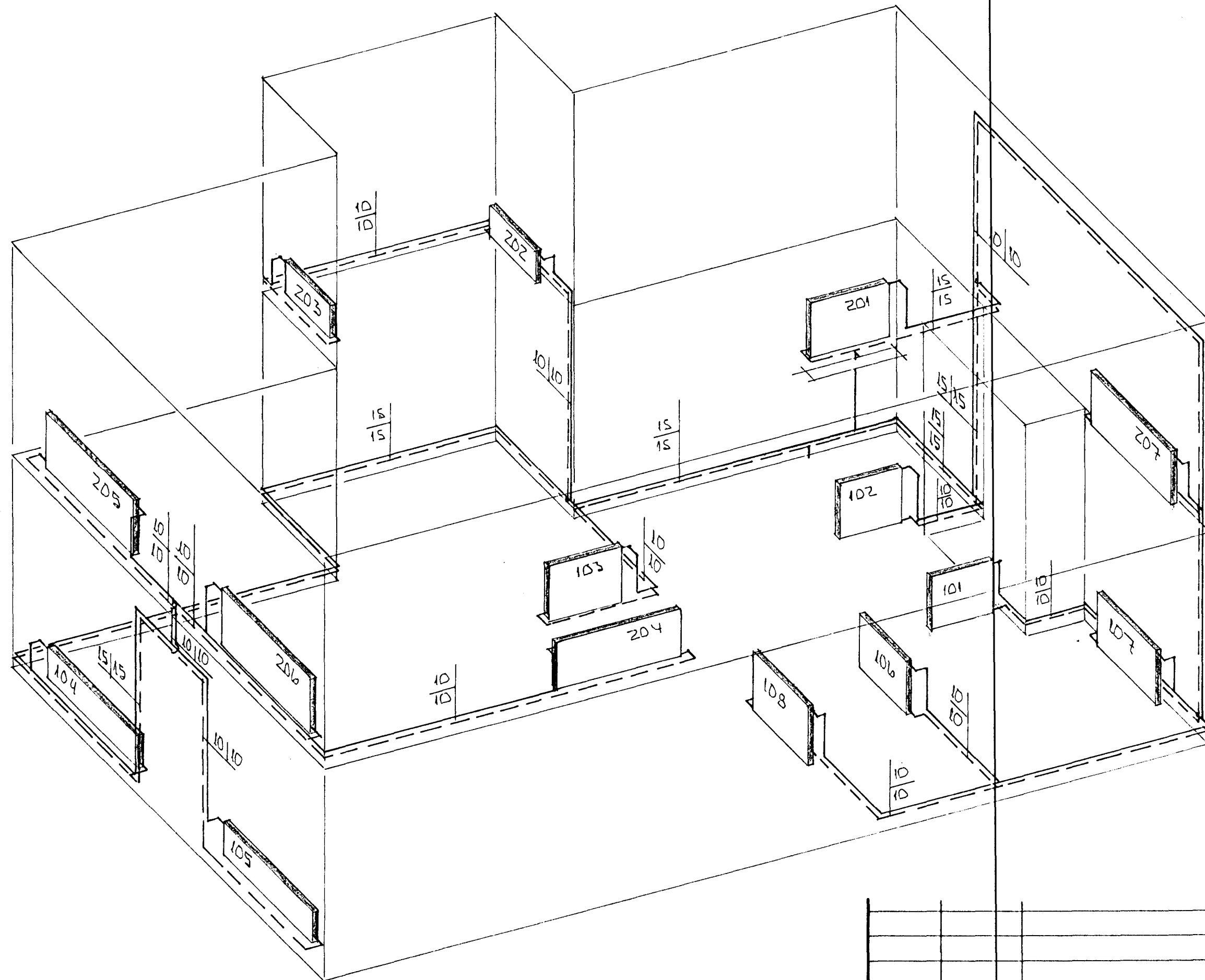
RÚMMYND HITALAGNA • 1:50
