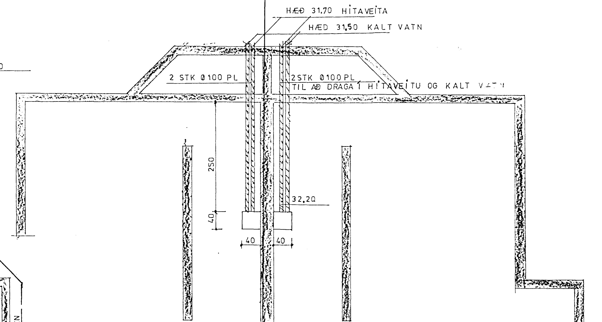
LAGNIR TIL AÐ DRAGA Í HITAVEITU OG KALT VATN M: 1:50
