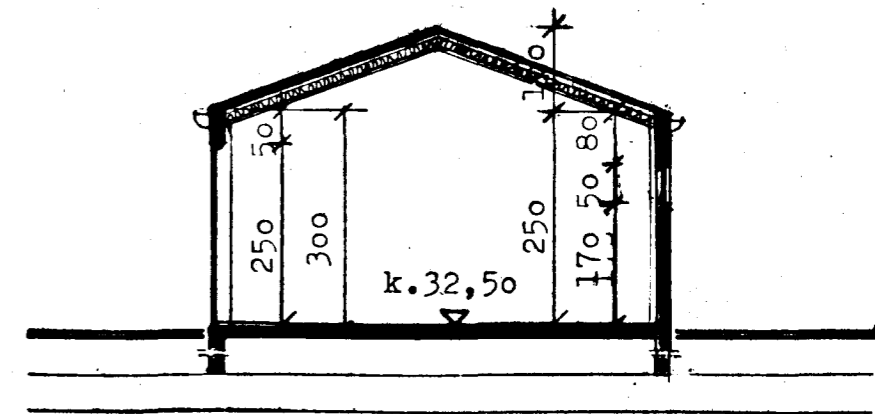
Þverskurður vestur-austur
