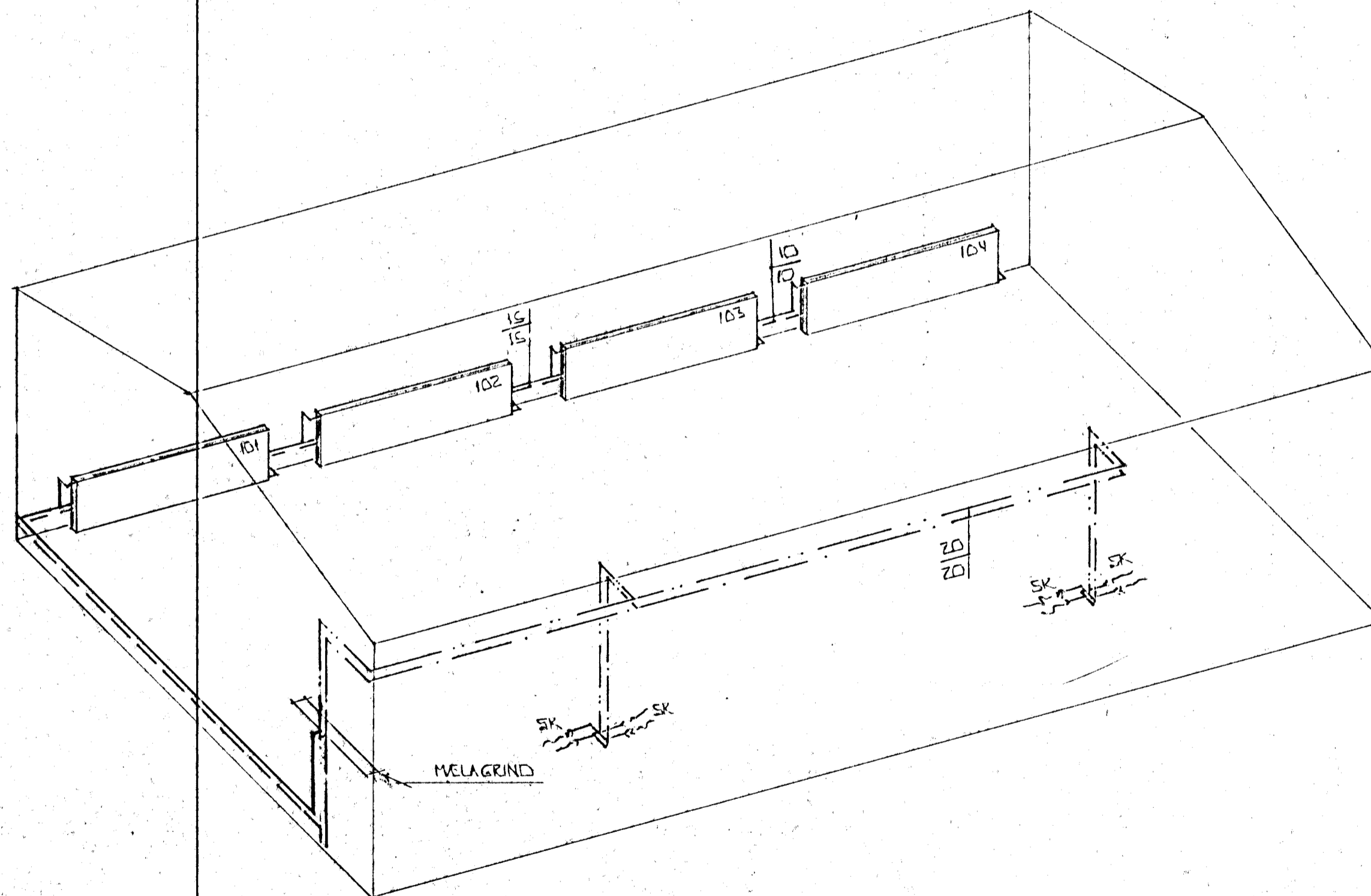
RÚMMYND LAGNA 1:50
