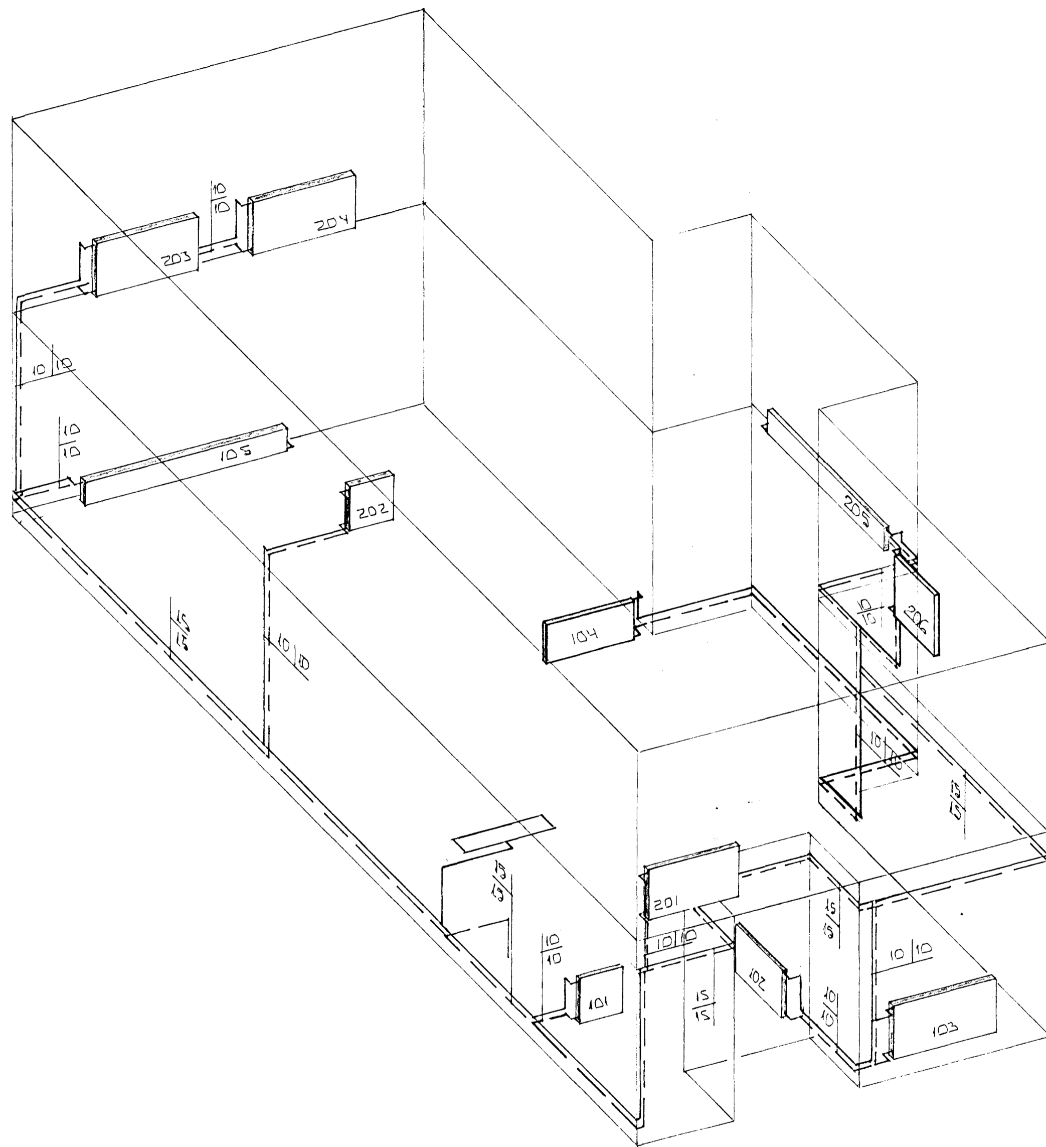
RÚMMYND HITALAGNA 1:50
