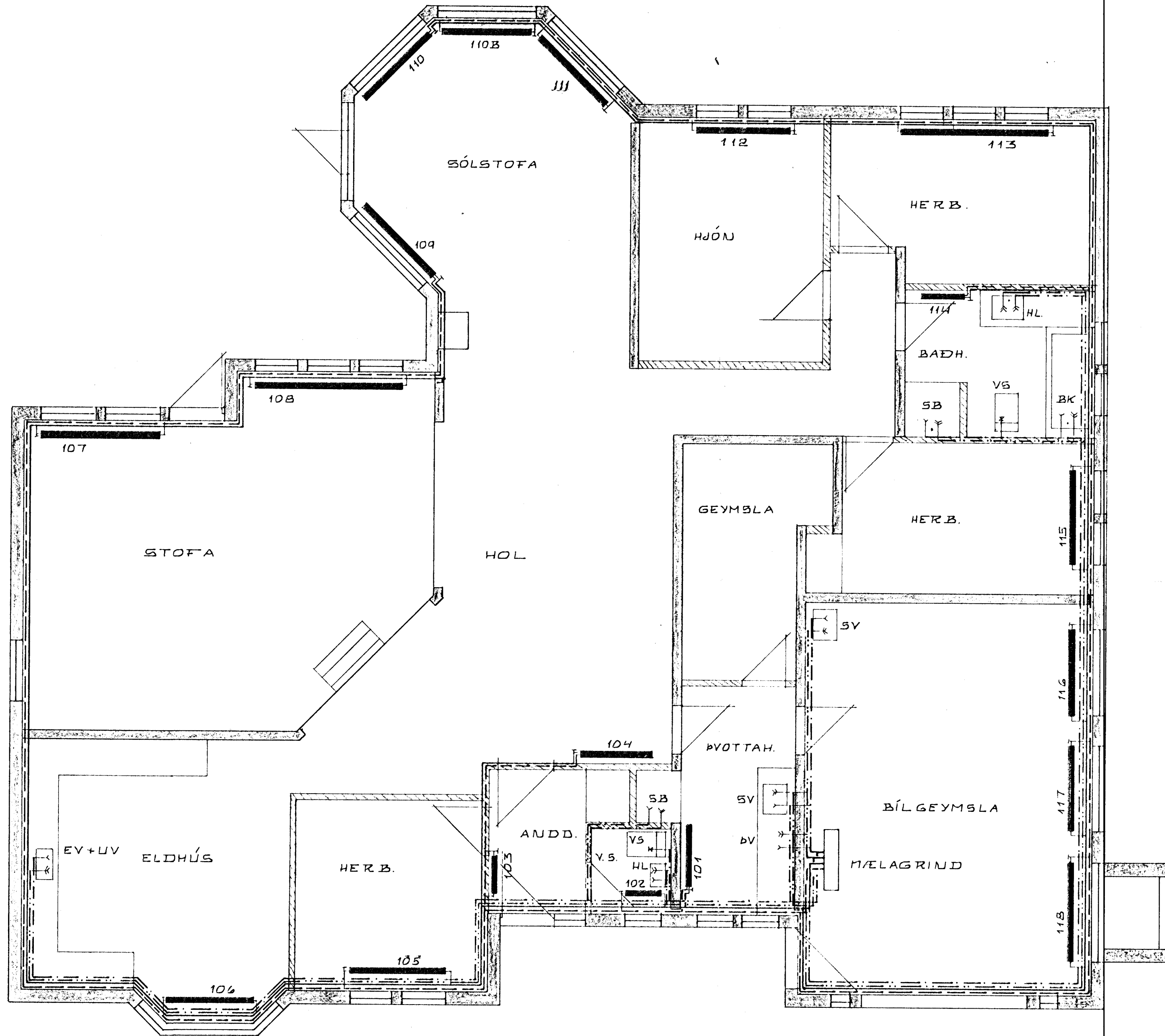
GRUNNMYND 1:50
