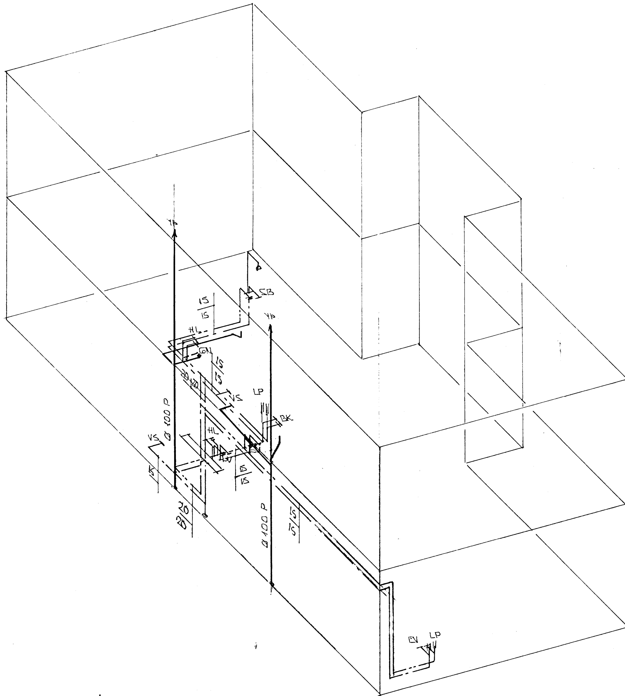
RÚMMYND VATNSLAGNA 1:50
