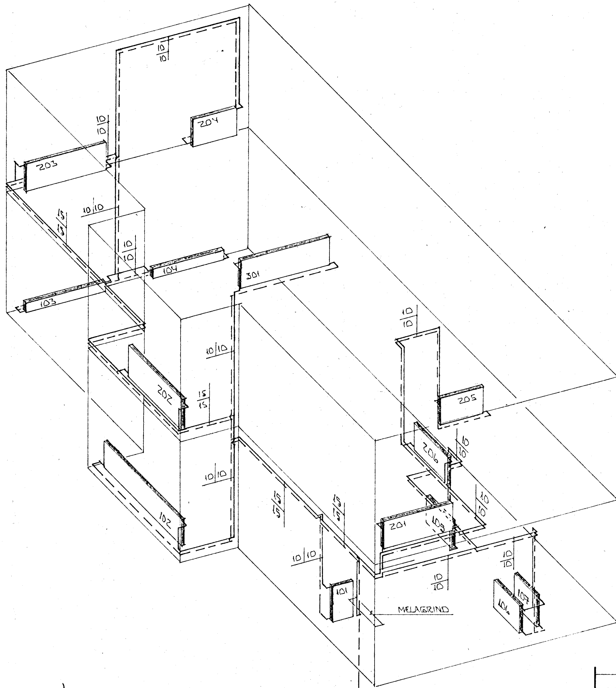
RÜMMYND HITALAGNA. 1:50
