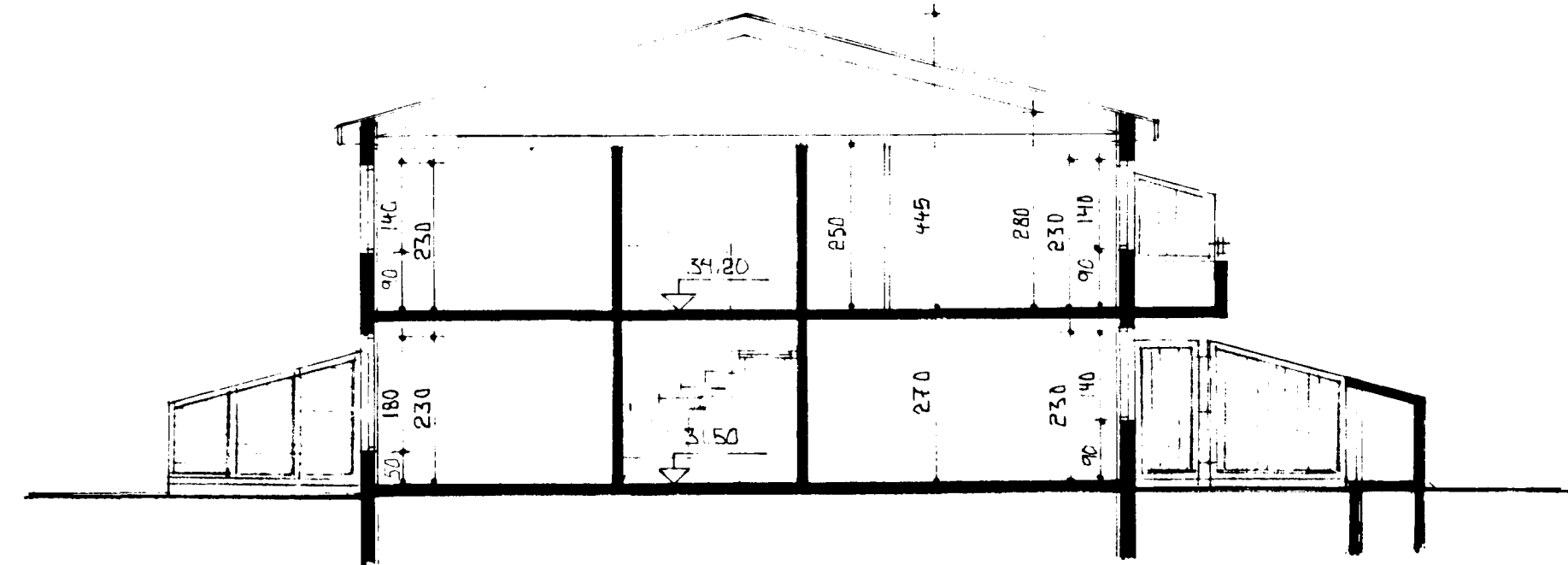
SNID M.1:100
