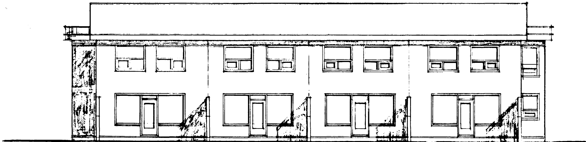
NORÐUR M.1:100
