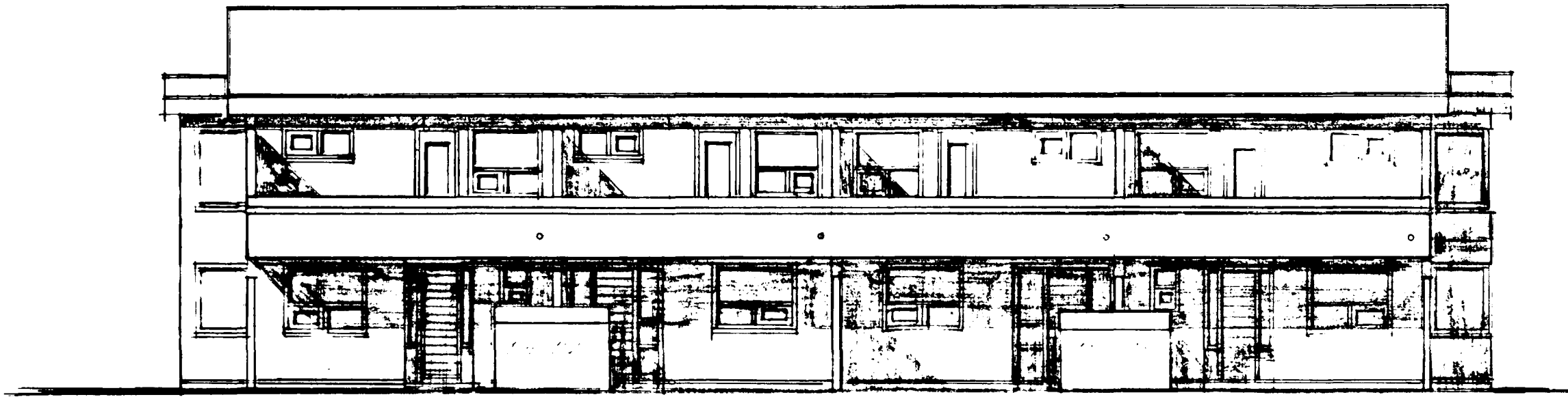
SUÐUR M.1:100
