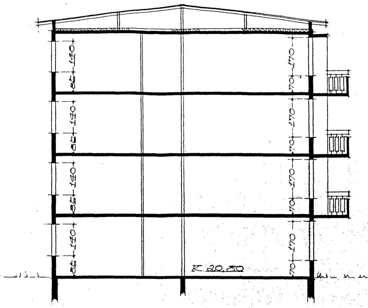
SKURÐUR B-B
