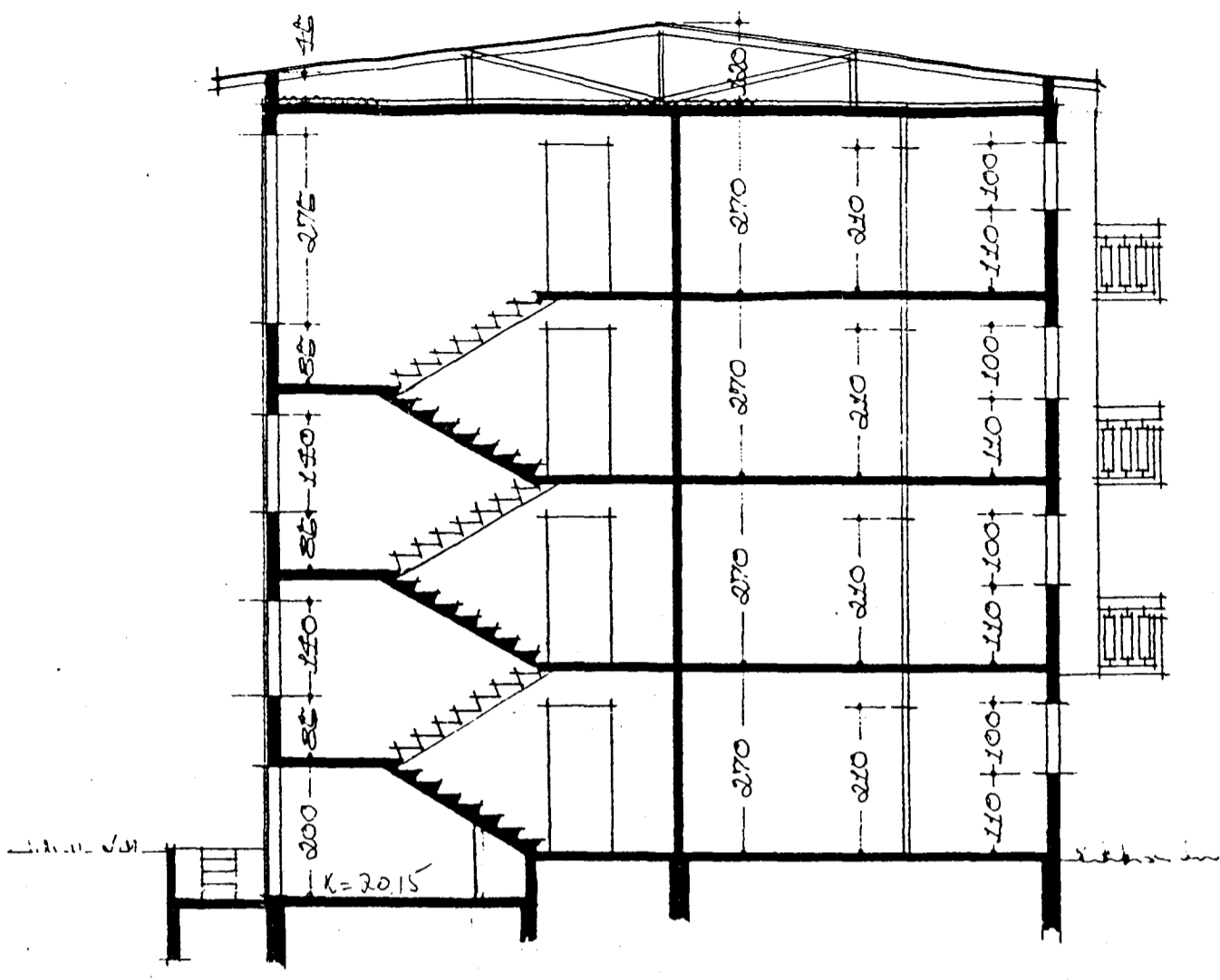
SKURÐUR A-A
