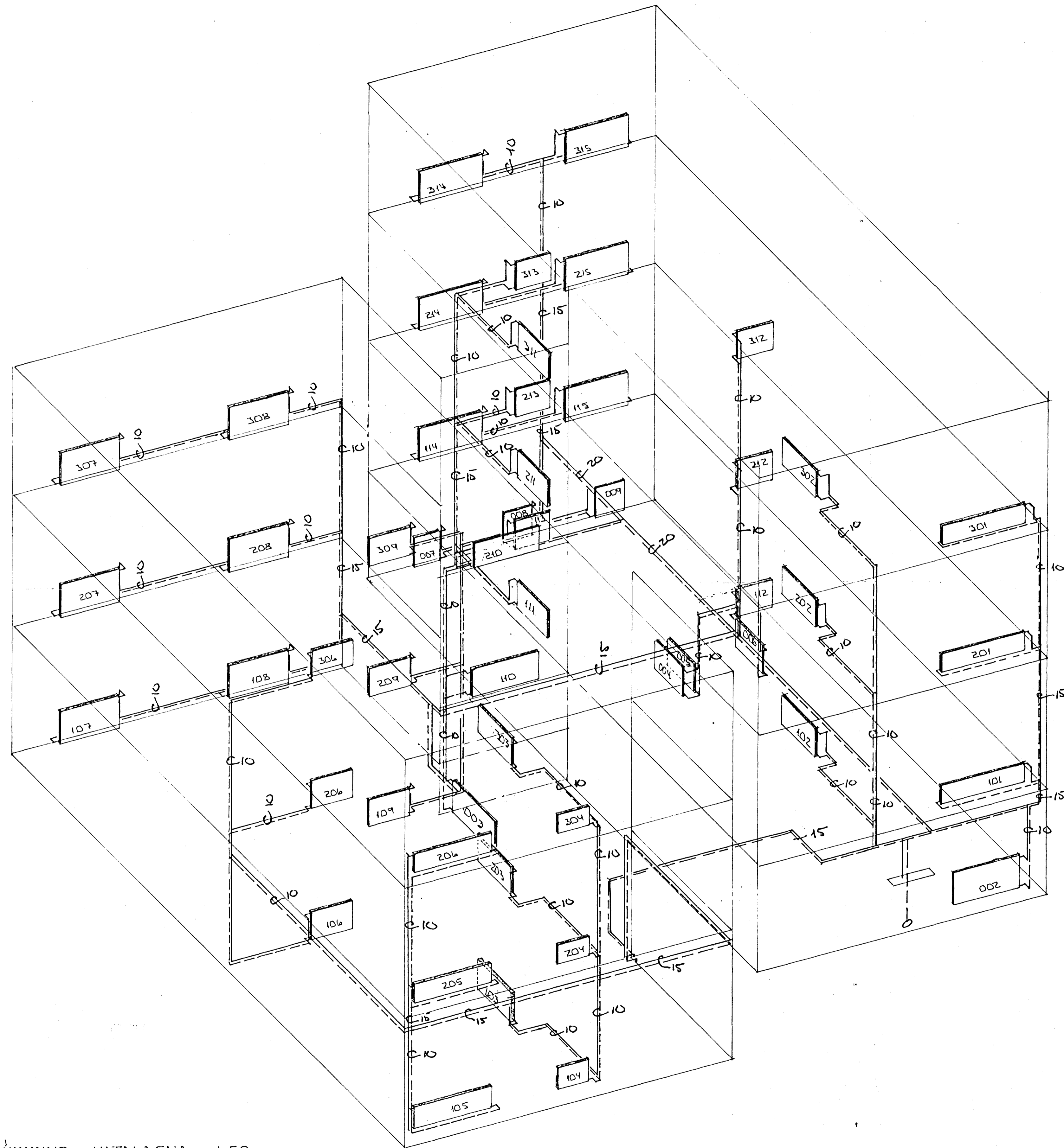
RÚMMYND HITALAGNA 1:50
