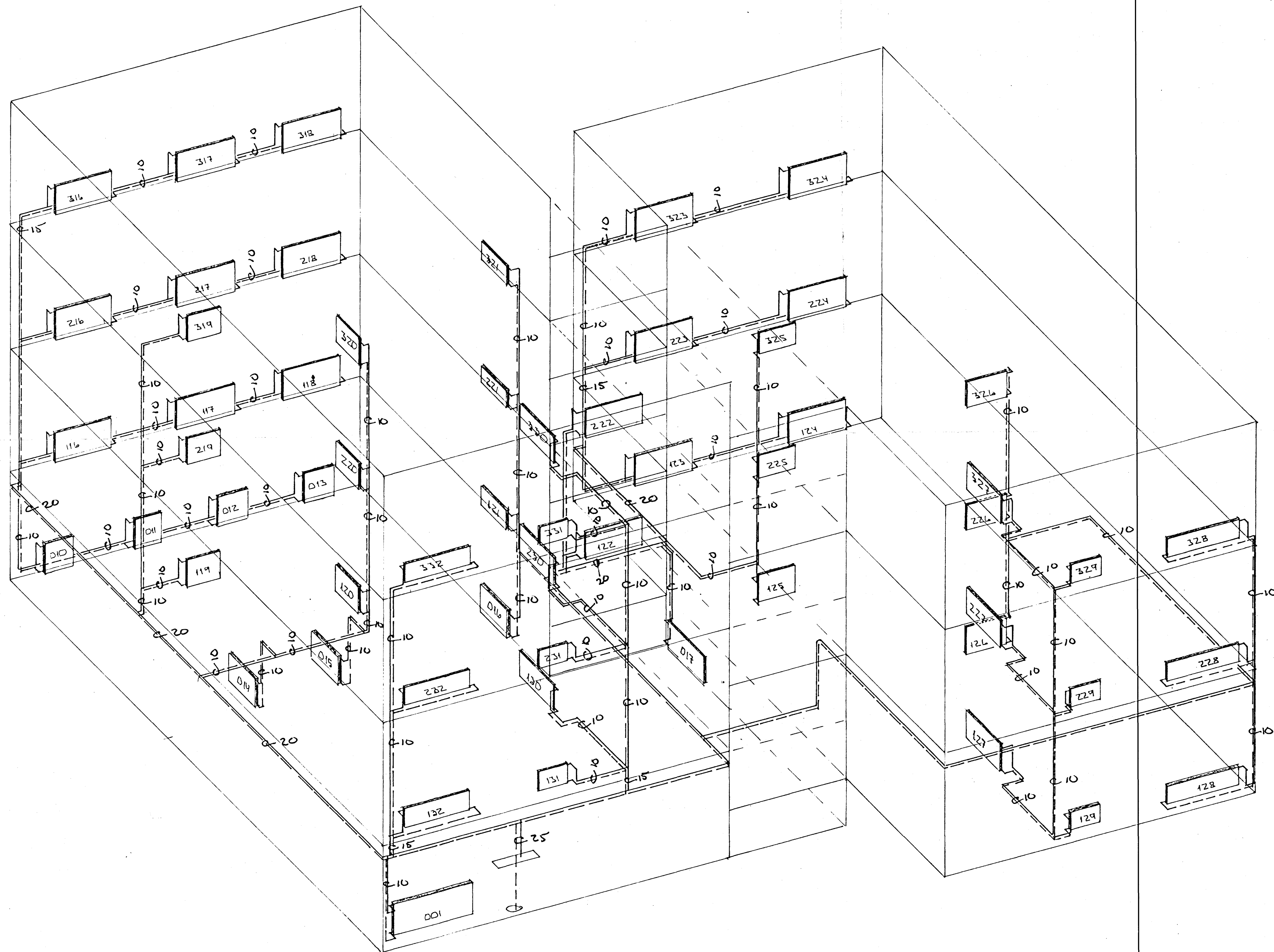
RÚMMYND HITALAGNA 1:50
