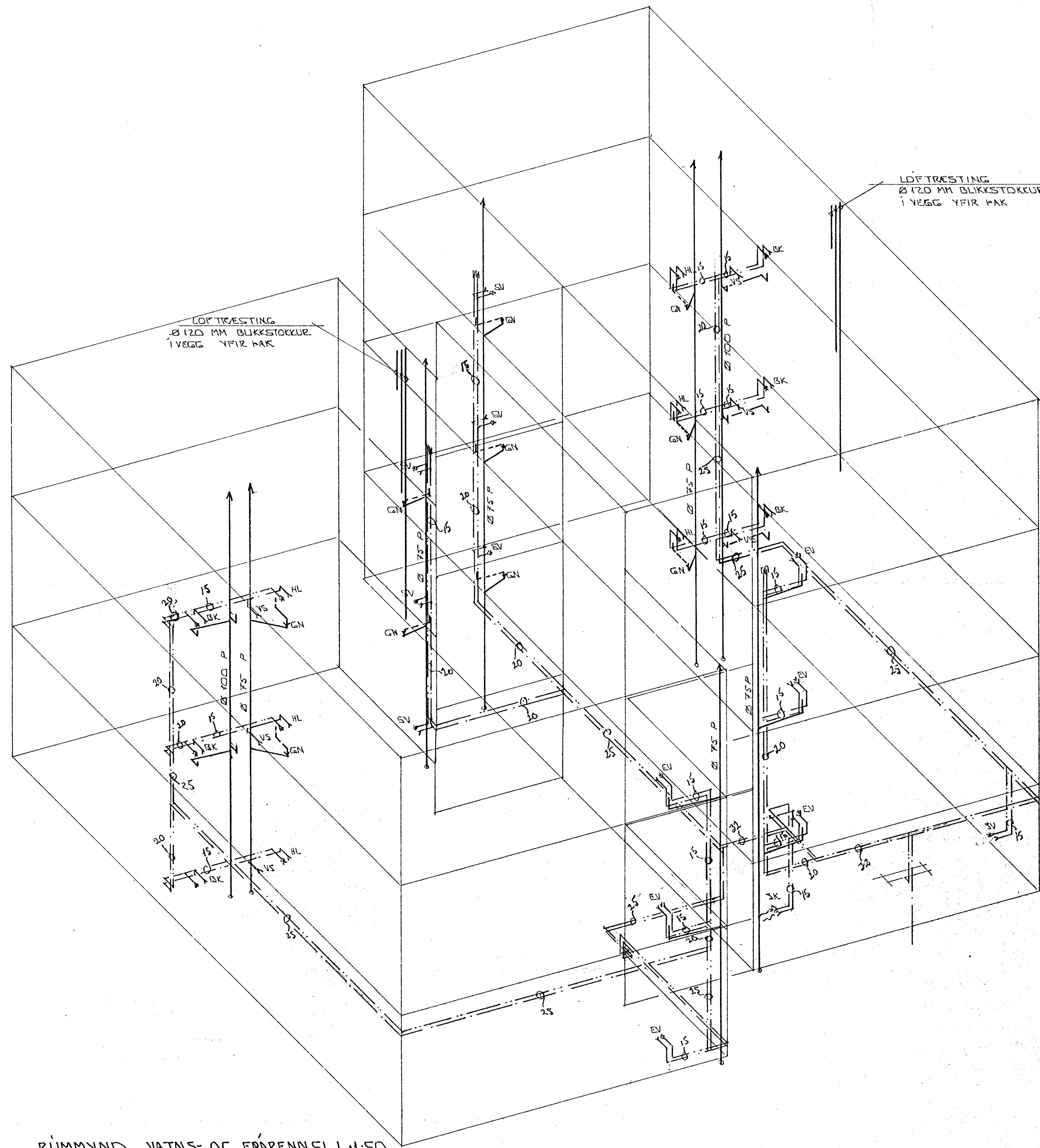
RÚMMYND VATNS- OG FRÆRENNSL.L.1:50
