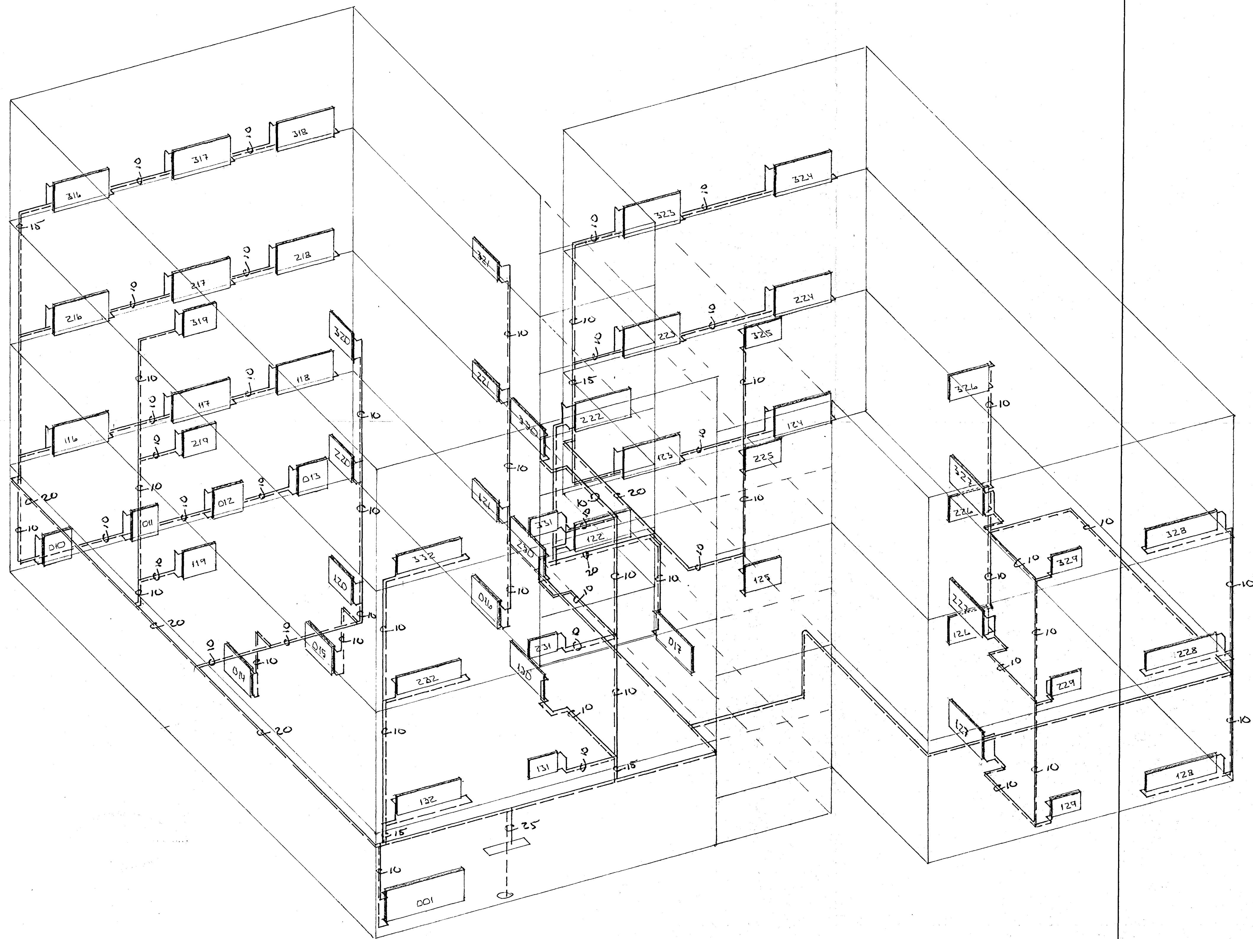
RÚMMYND HITALAGNA 1:50
