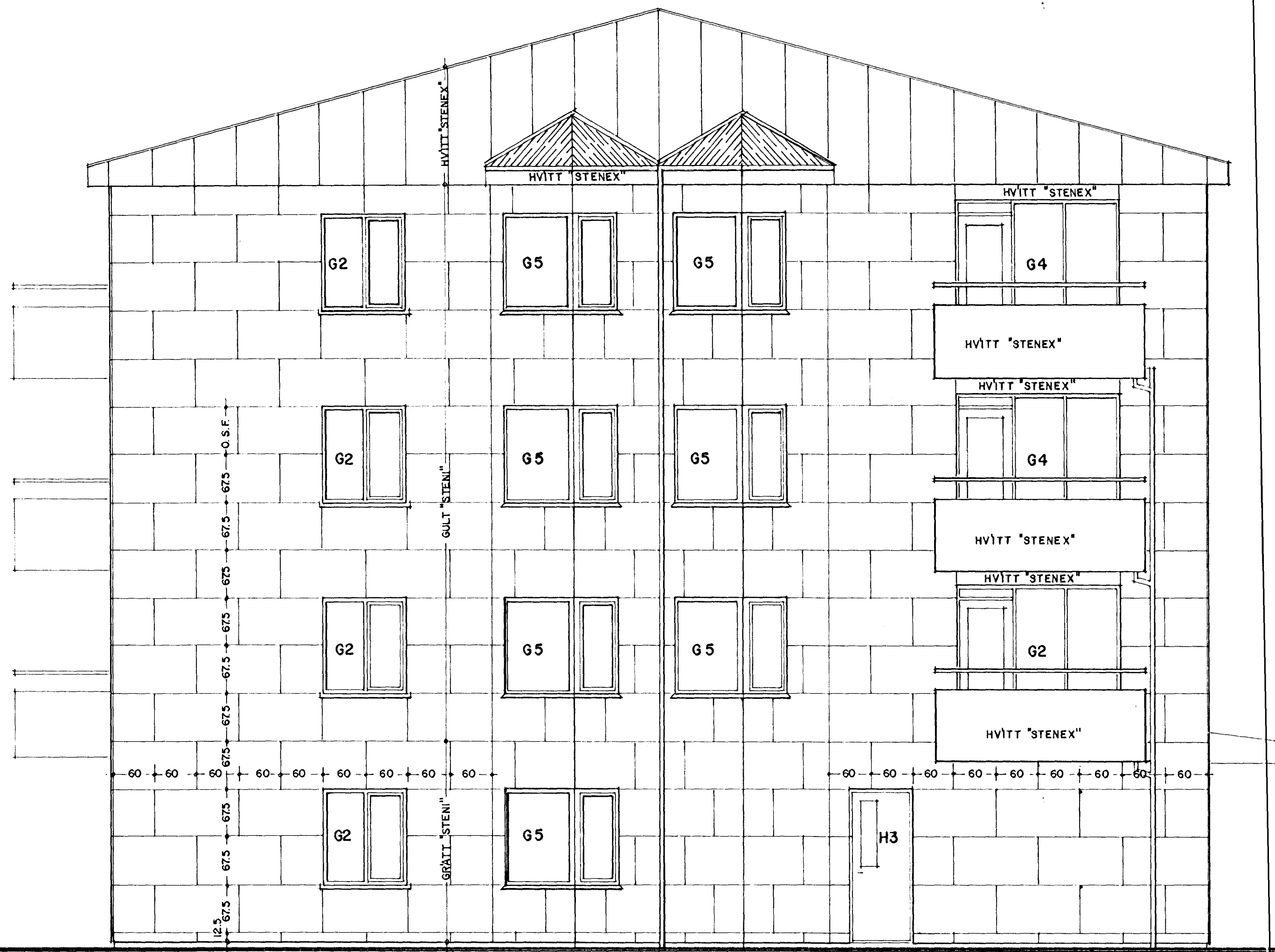
ÚTLIT AUSTUR 1:50
