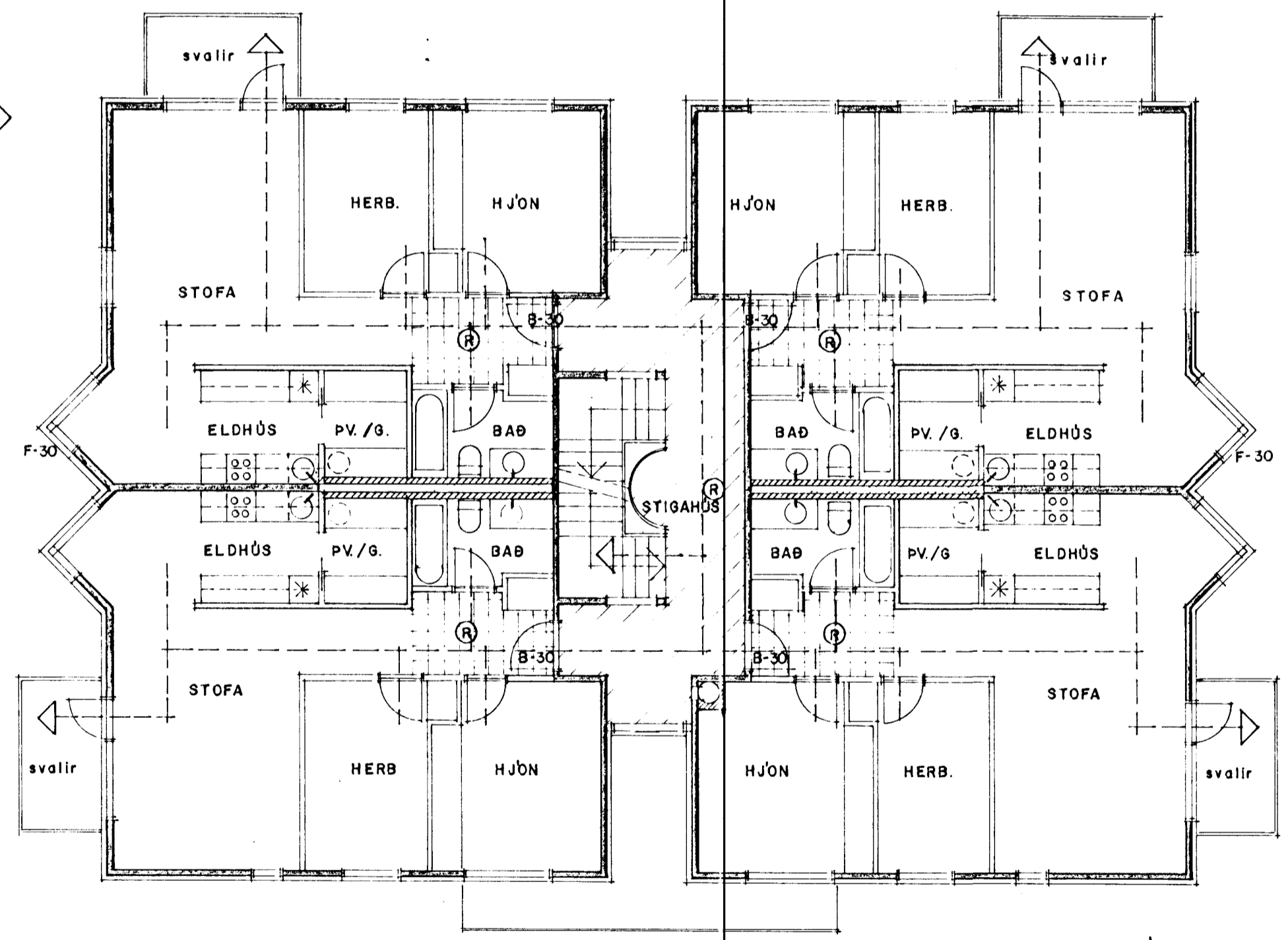
GRUNNMYND 2.-4. H/ÆÐ 1:100
