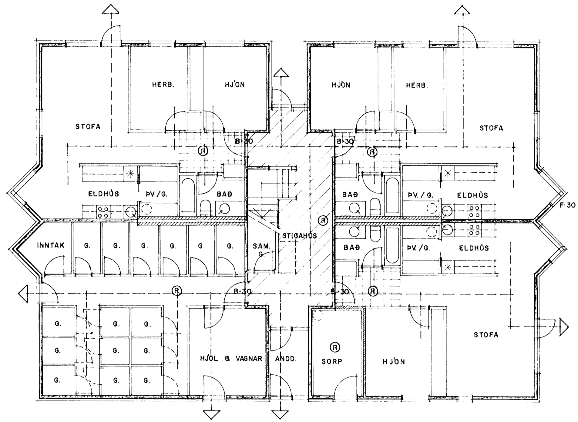
GRUNNMYND 1. H/ÆÐ 1:100
