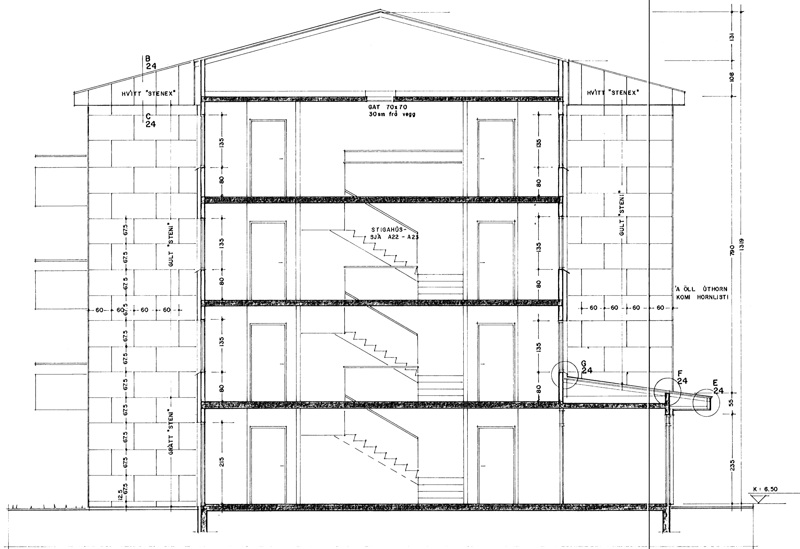
SNEIÐING C - C 1:50
