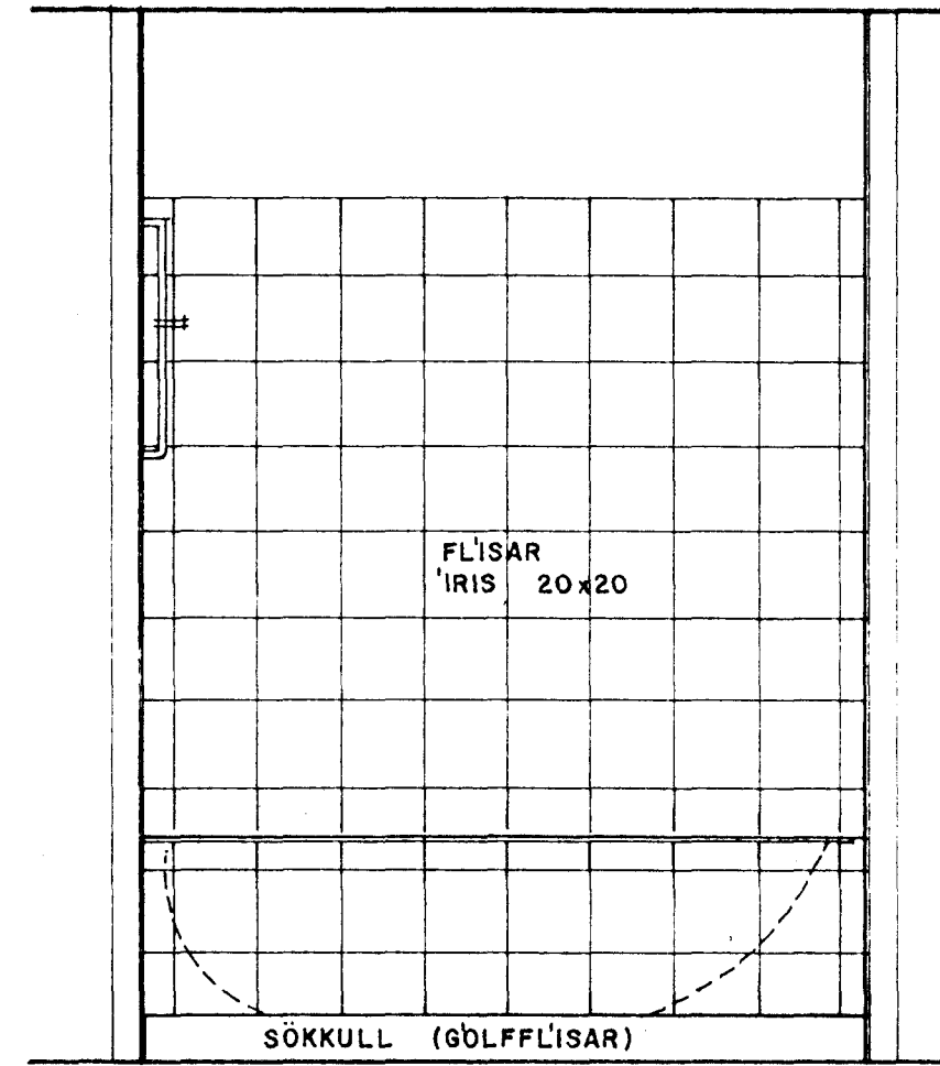
HLIÐARMYND 1:20
