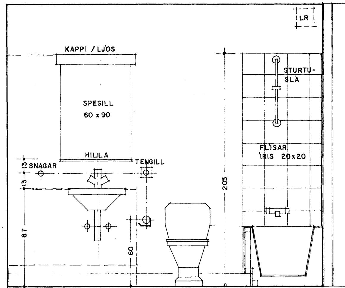
HLIÐARMYND 1:20
