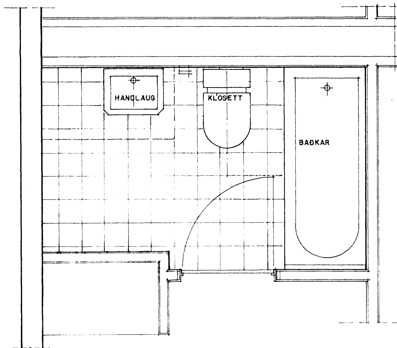
GRUNNMYND 1:20
