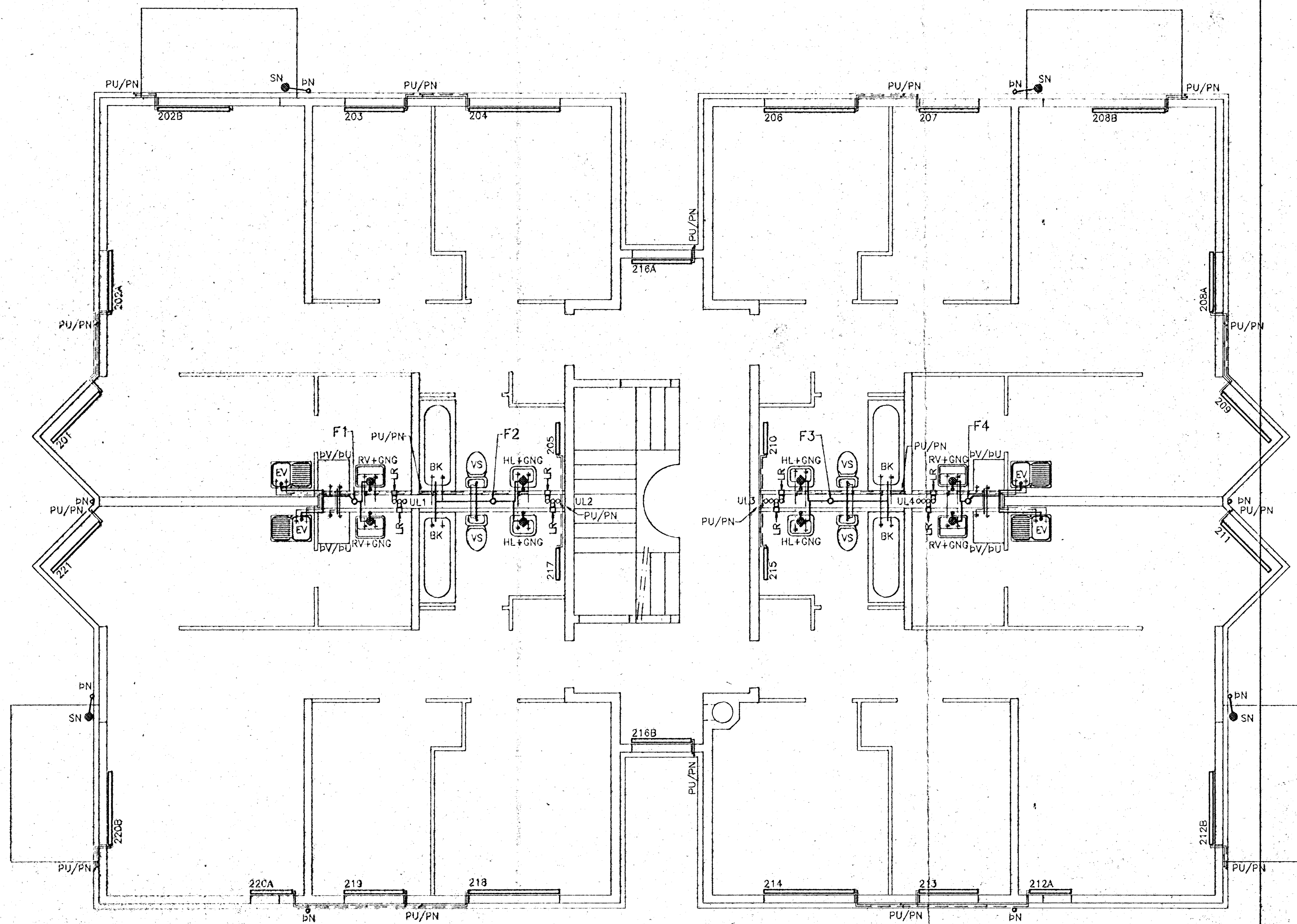
GRUNNMYND 2. HÆÐAR 1:50
