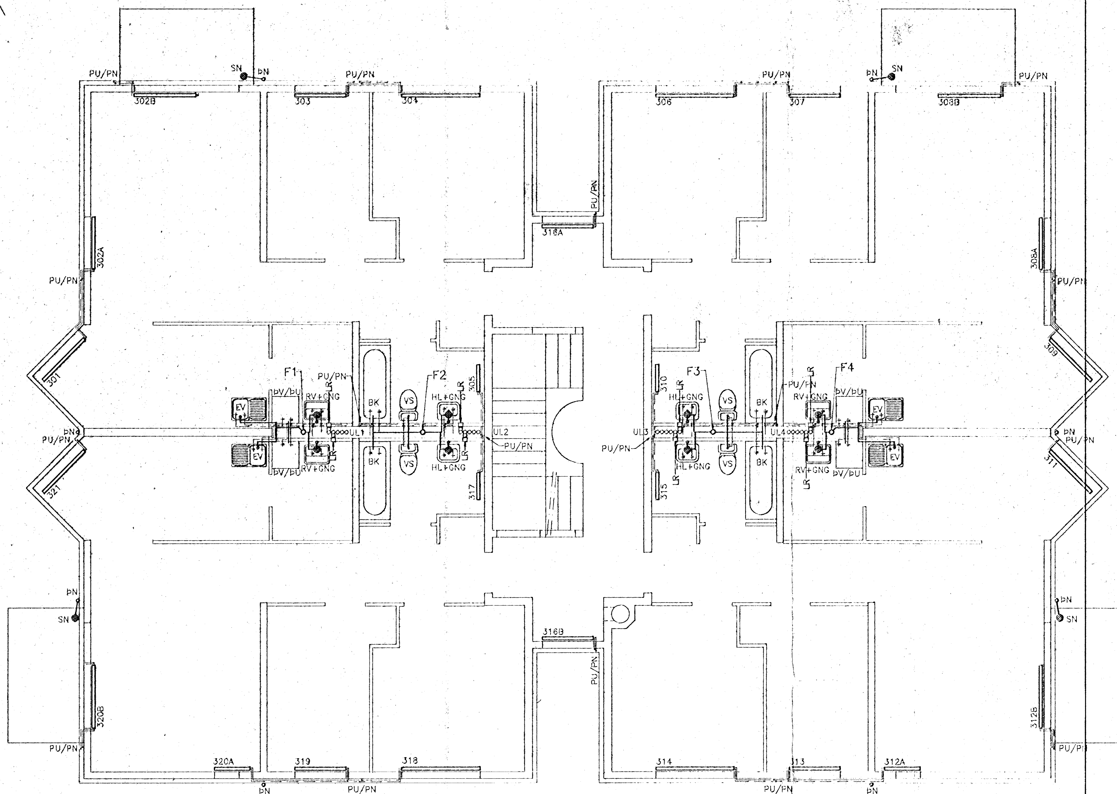
GRUNNMYND 3. HÆÐAR 1:50
