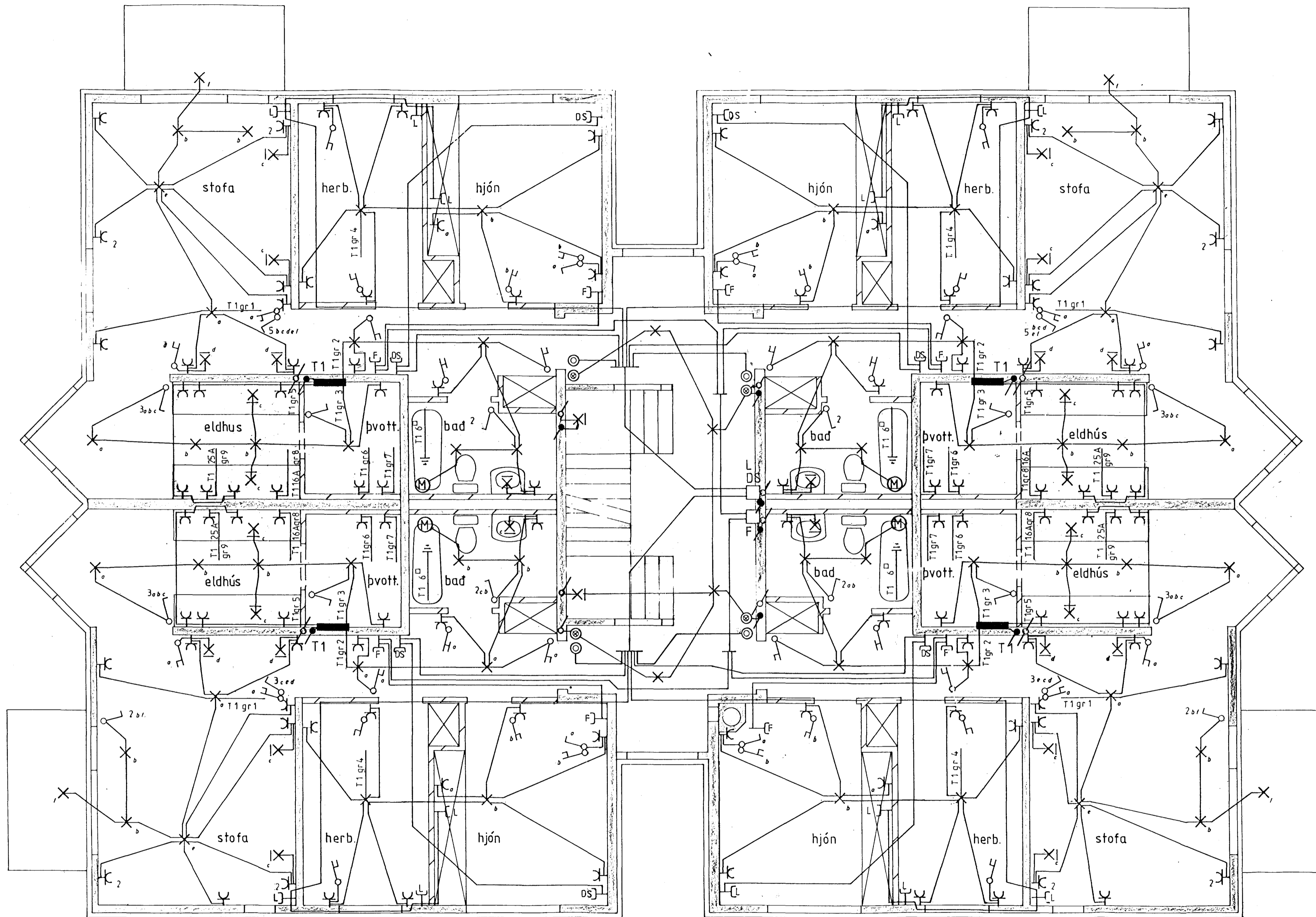
Grunmynd 2 hæð mkv 1:50
