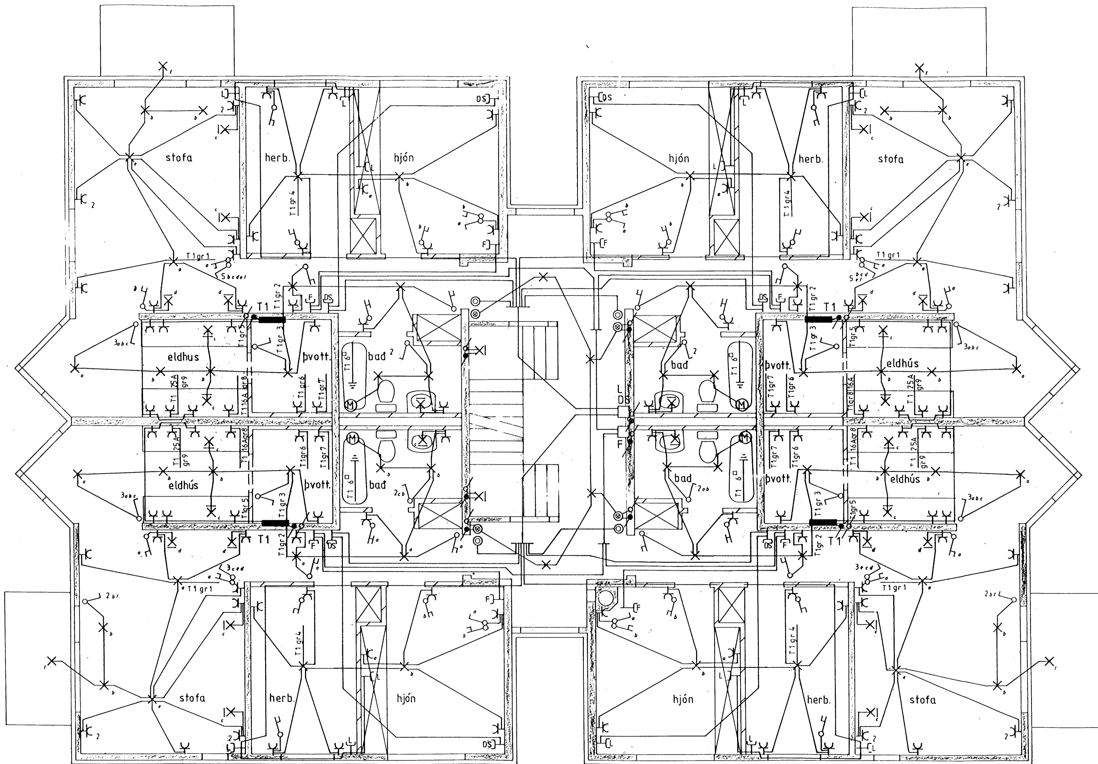
Grunnmynd 3 hæð mkv 1:50
