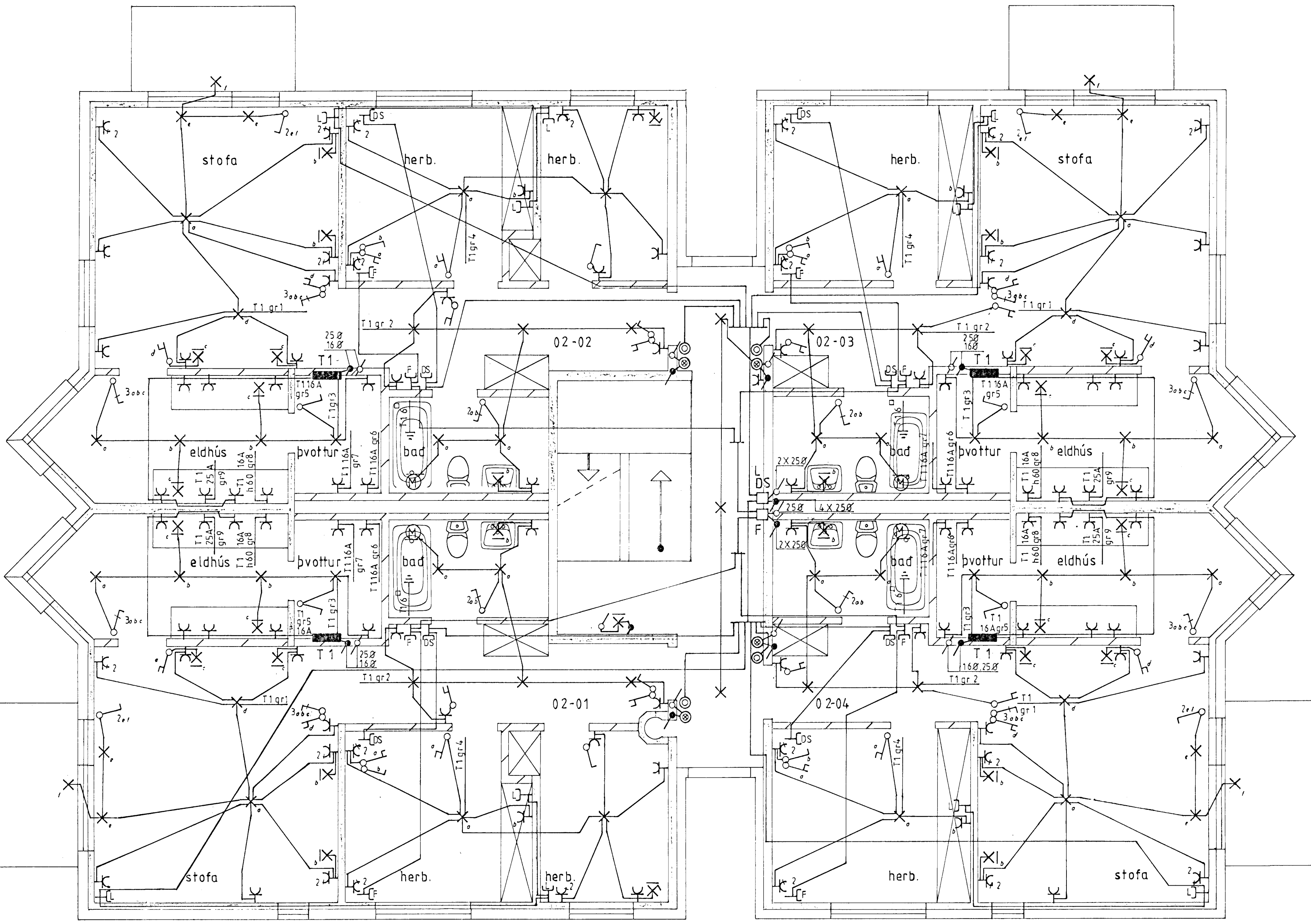
Grunnmynd mkv. 1:50
