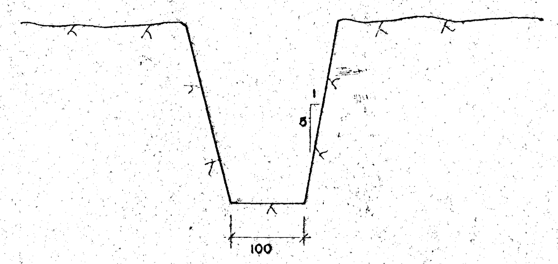
DVERSNIÐ Í SPRENGDAN LAGNASKURÐ
