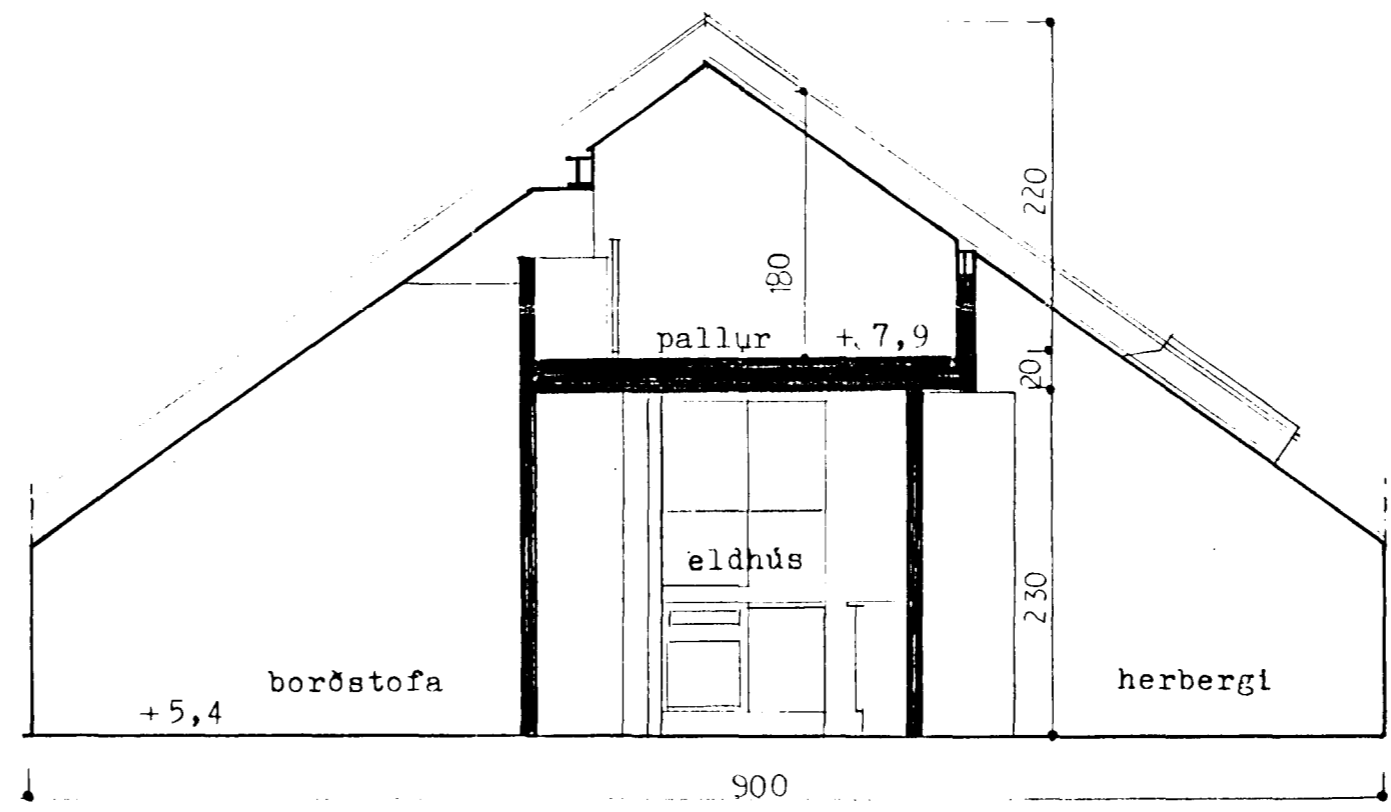
Suðurgata 17 2.hæð Skurður 1/50
