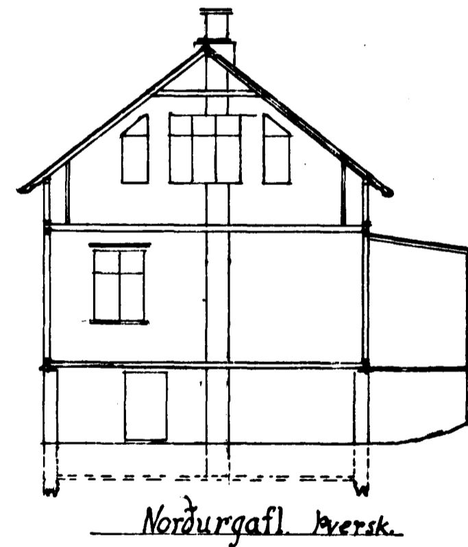
Máli kv 1.100
