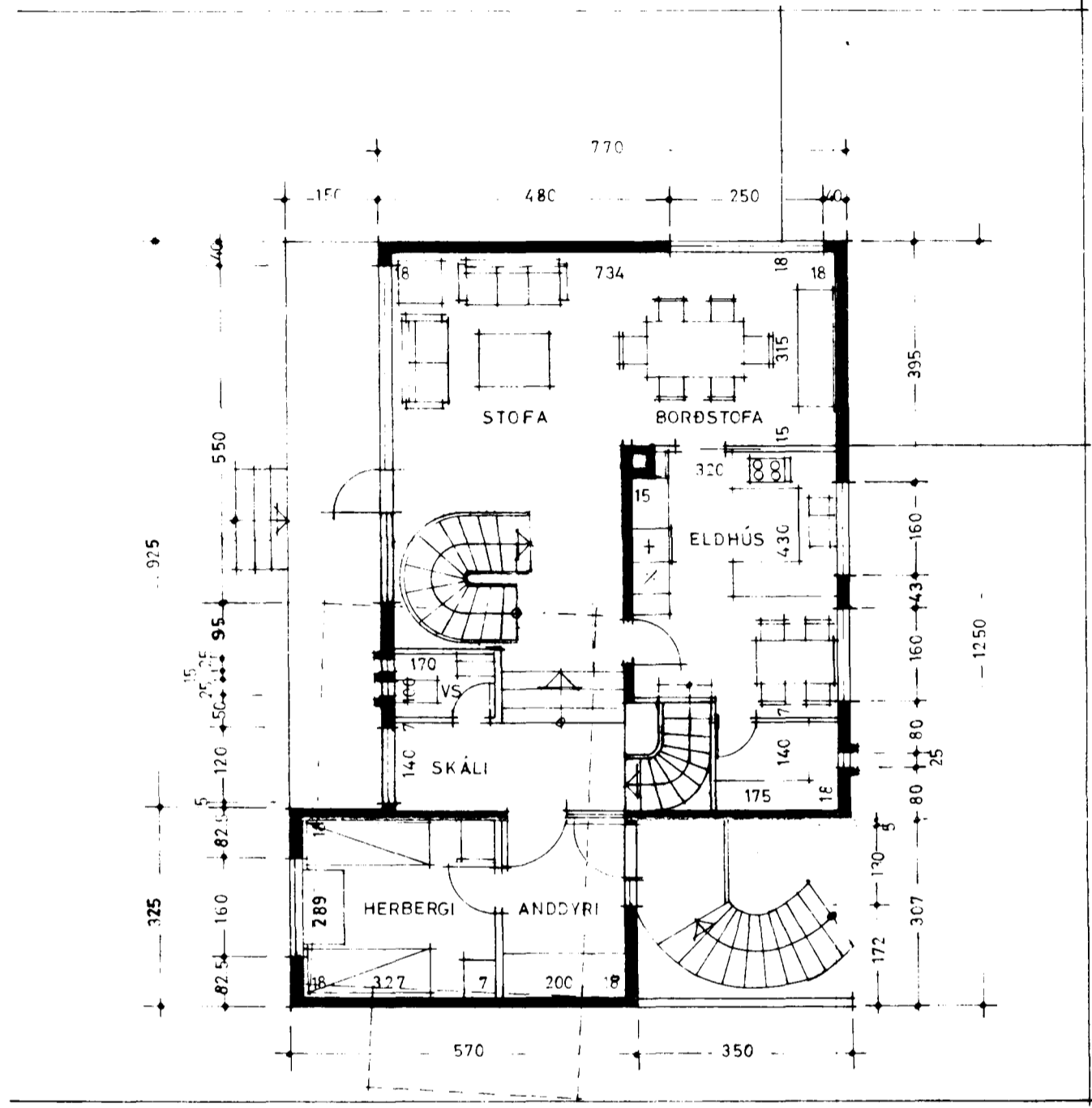
1. HÆÐ
