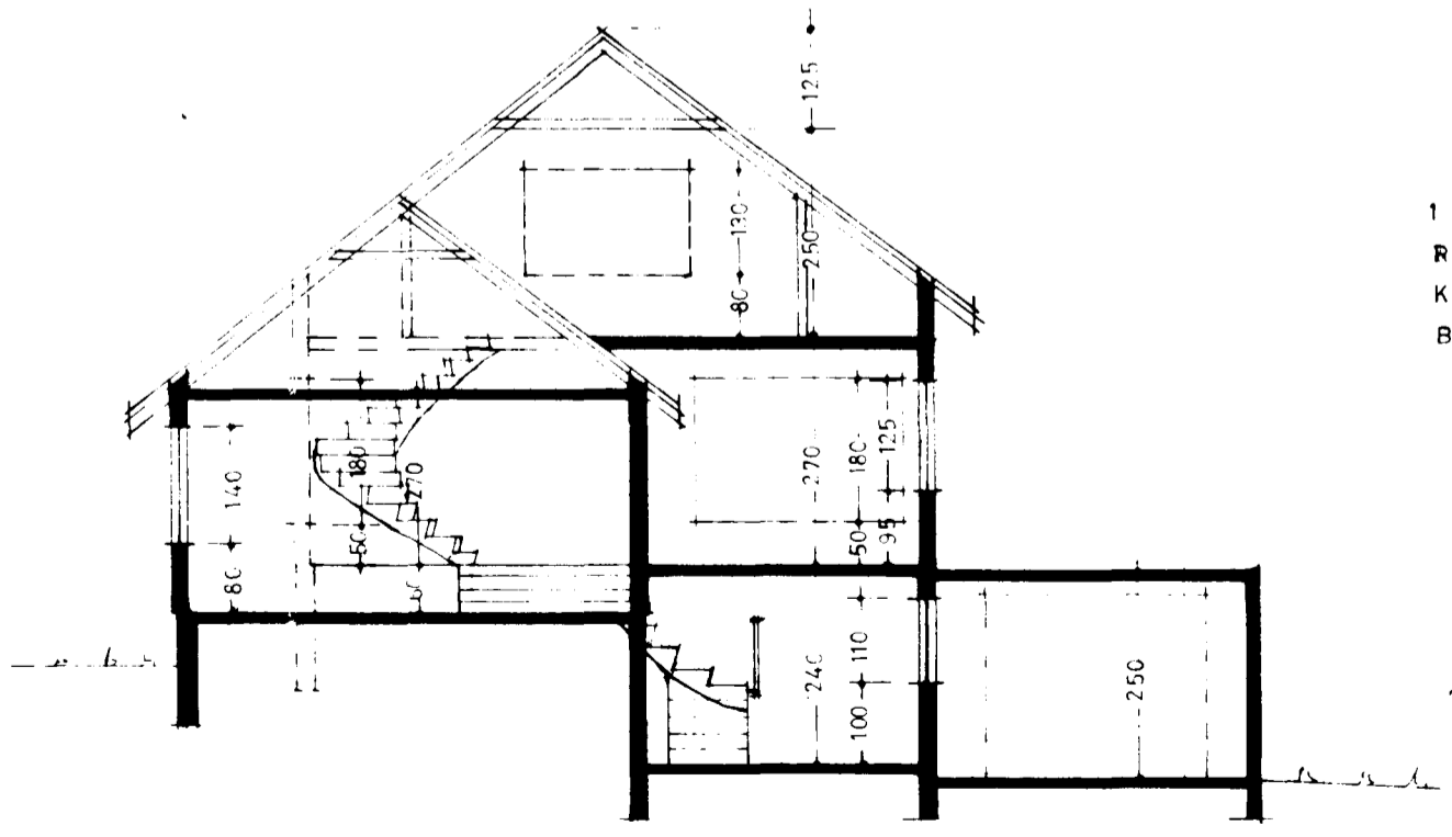
SNEIÐING
