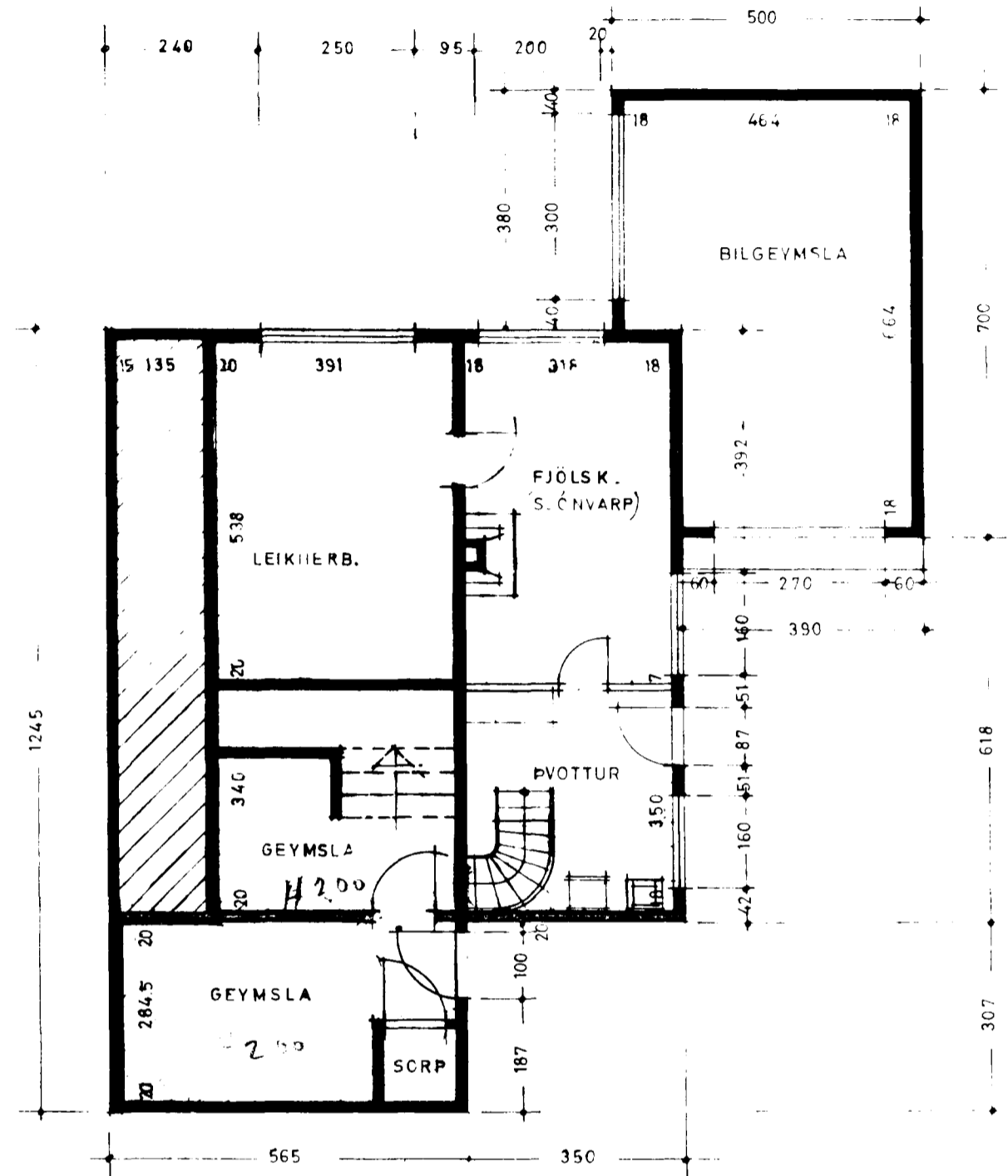
KJALLARI
