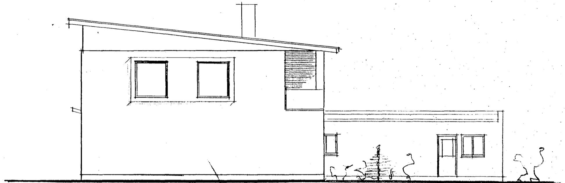
ÚTLIT NORÐUR HKV 1:100
