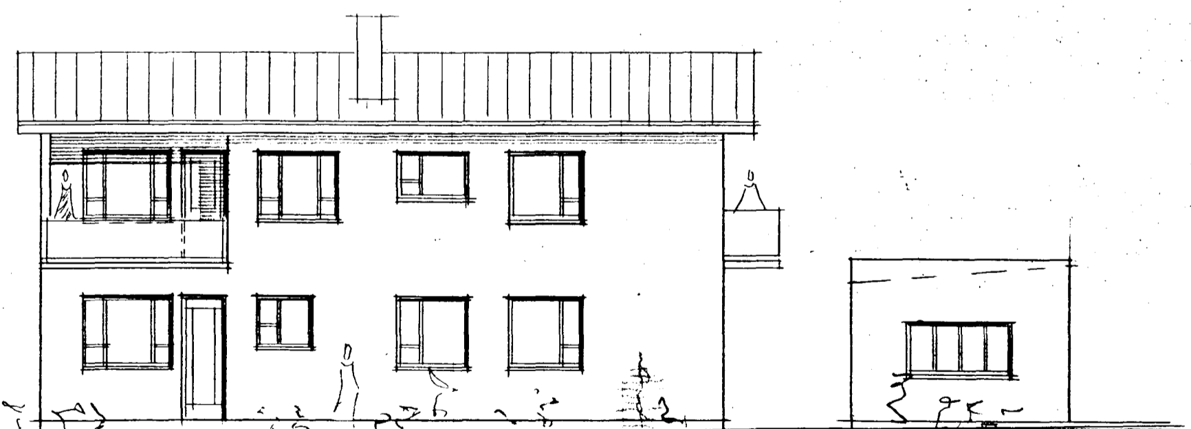
MHL 01 MHL 02 ÚTLIT VESTUR HKV 1:100
