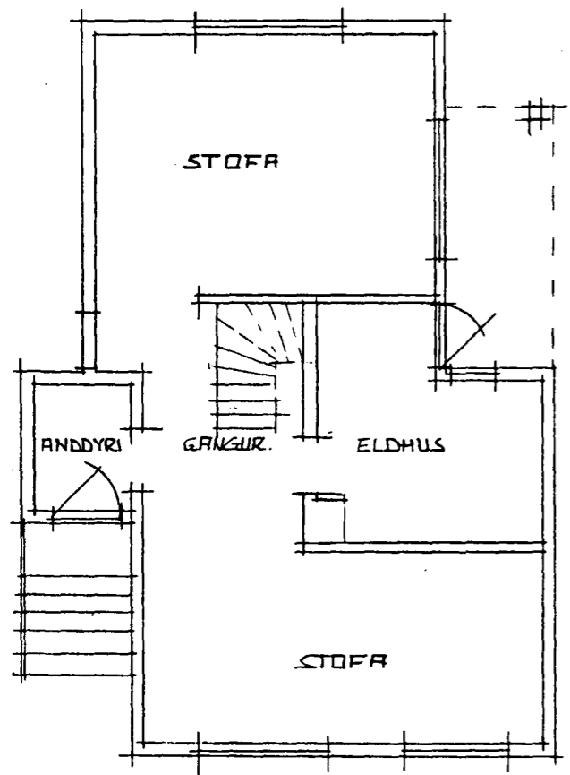
GRUNNMYND 1. HÉÐAR
