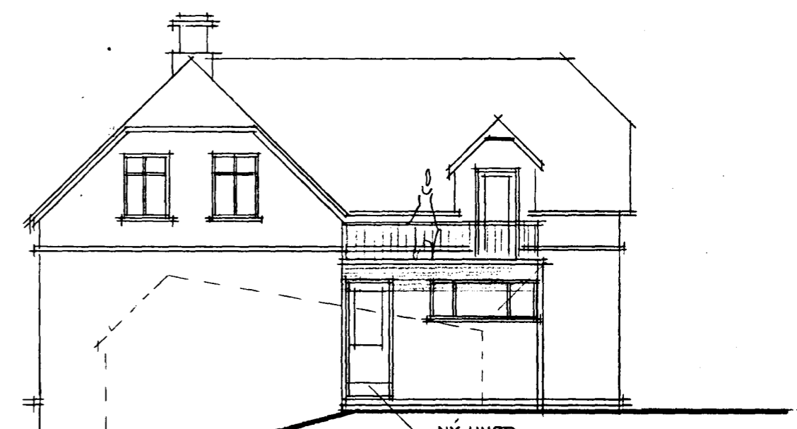
ÚTLIT VESTUR
