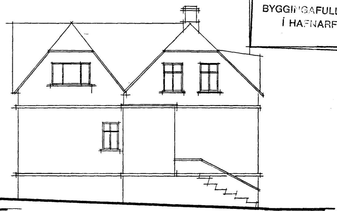
ÚTLIT AUSTUR
