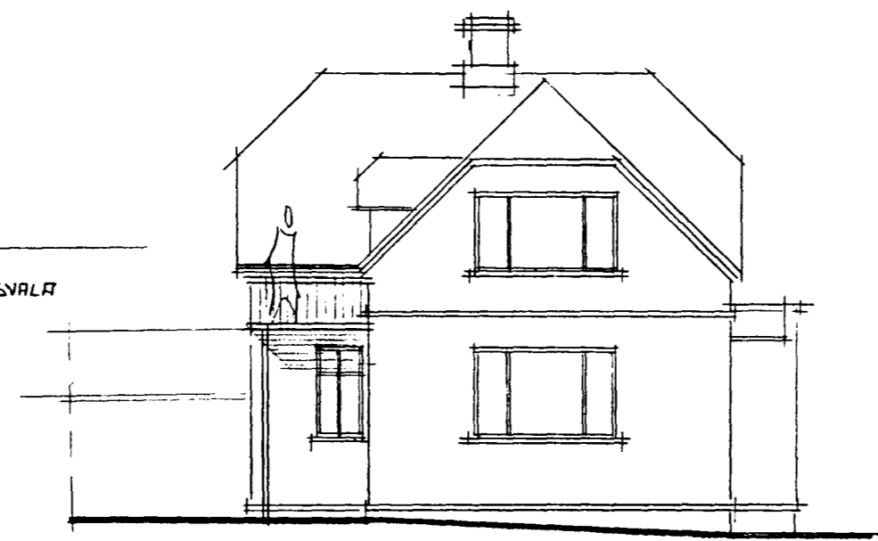
ÚTLIT SÚÐUR
