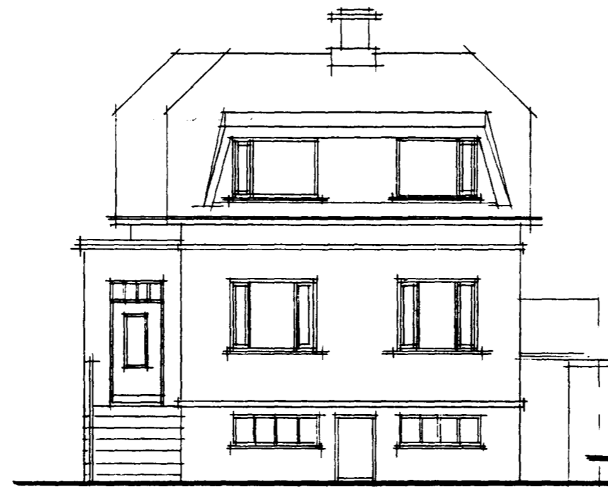
ÚTLIT NORÐUR
