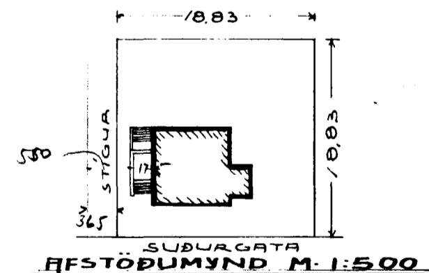
SUÐURGATA FESTOÐUMYND M-1:500
