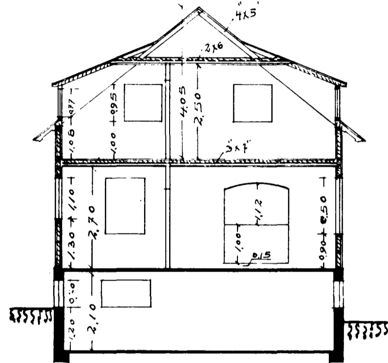
SKURÐUR A-B
