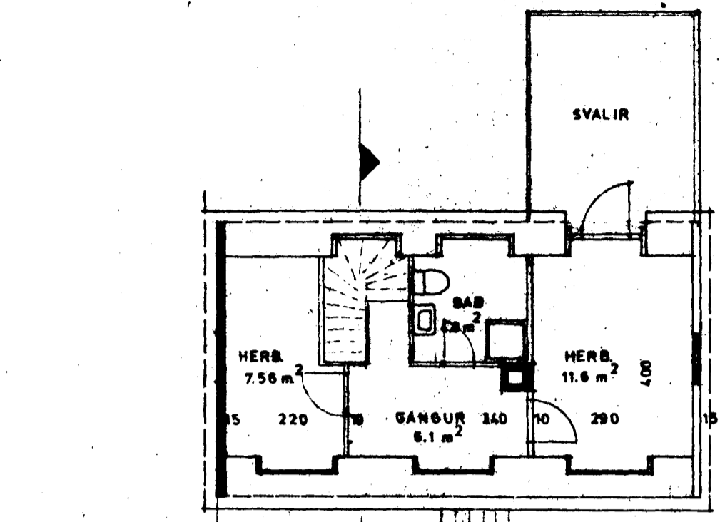
GRUNNMYND 2. HÆÐ
