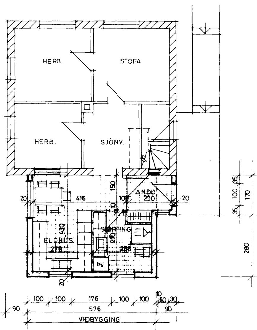
GRUNNMYND 1:100
