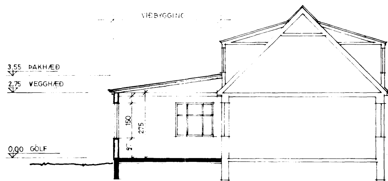
SNIÐ 1:100
