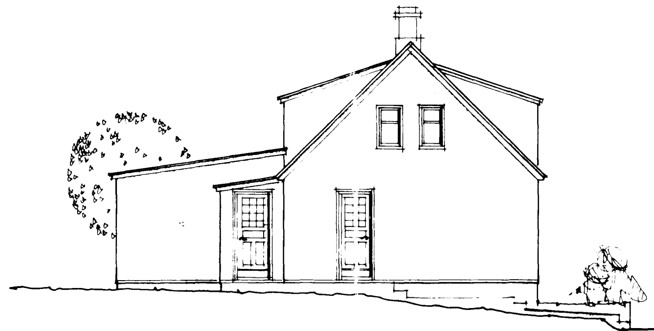
AUSTUR 1:100
