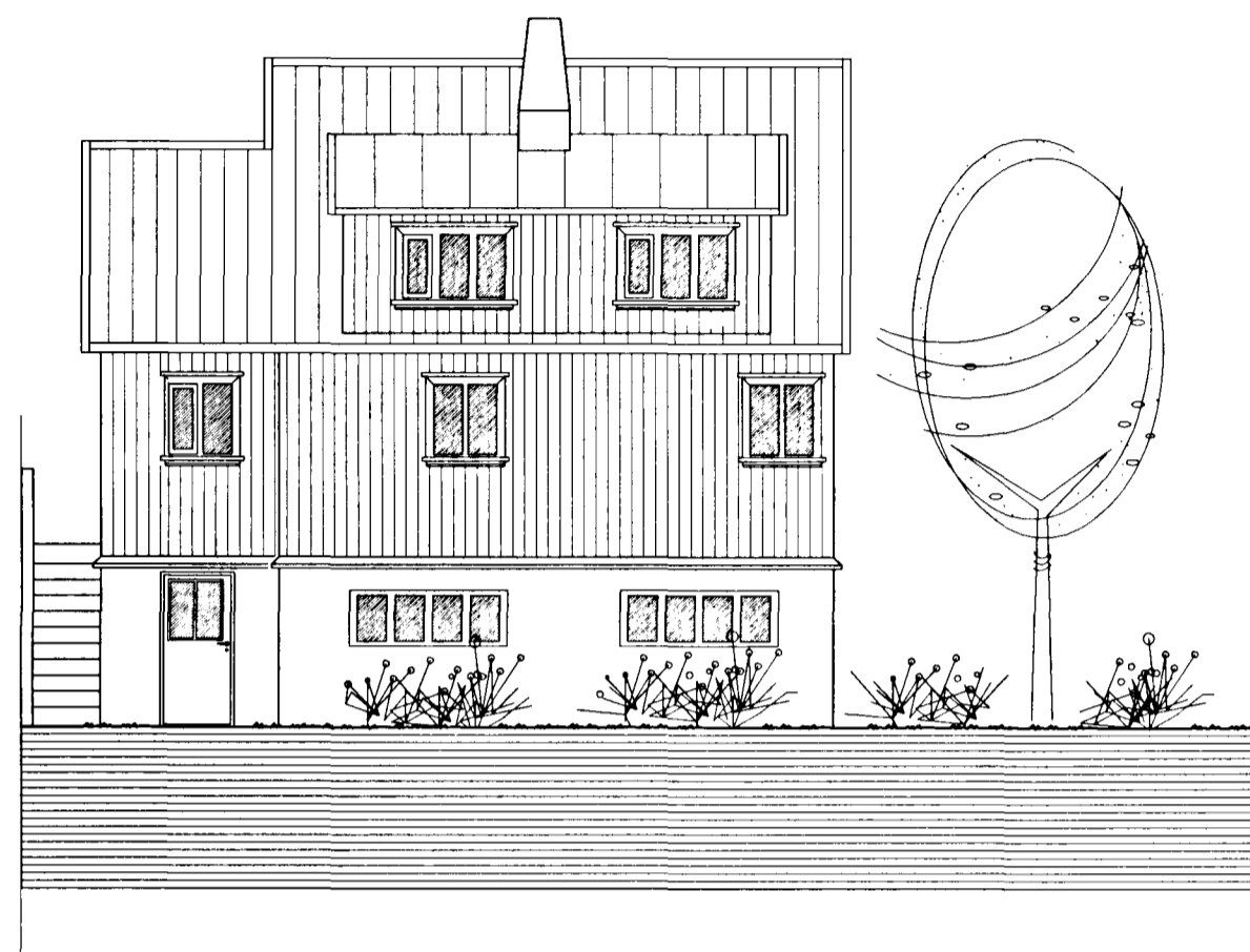
NORDVESTURHLID 1:100
