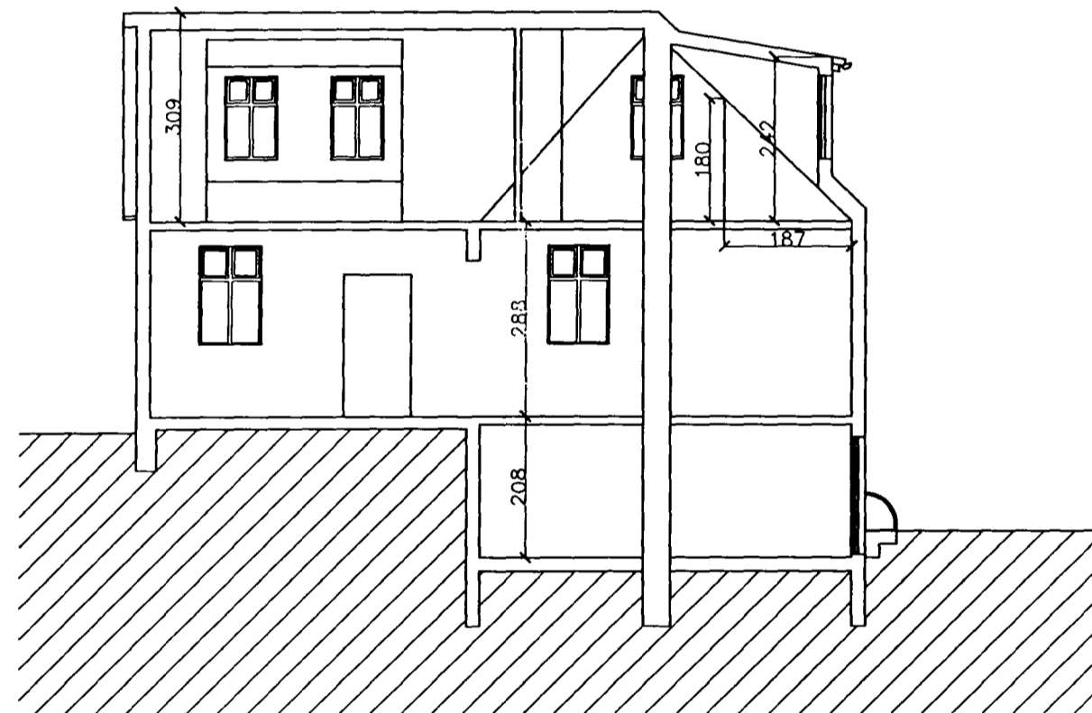
Snið B - B
