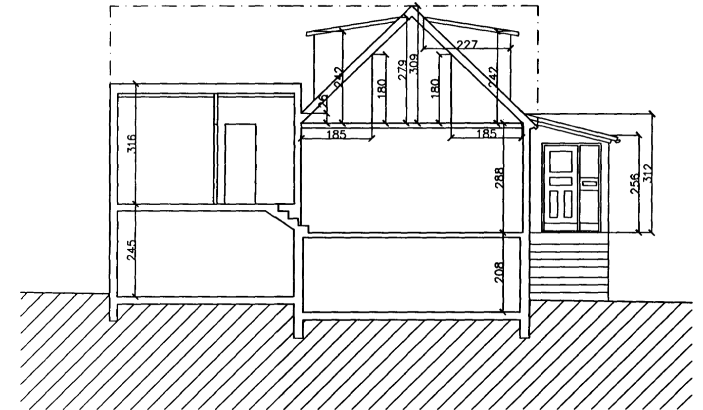
Snið C - C
