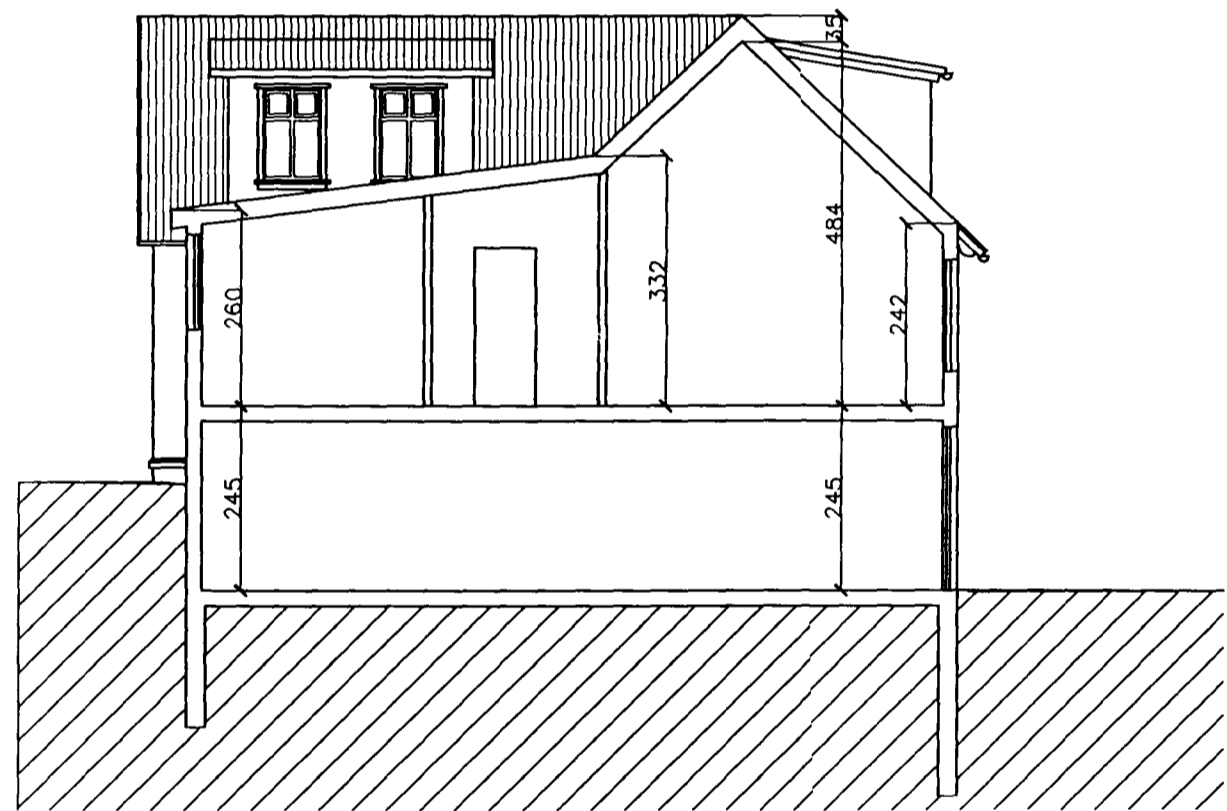
Snið A - A
