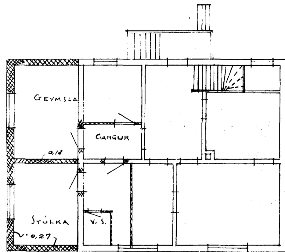
KJALLARI.
