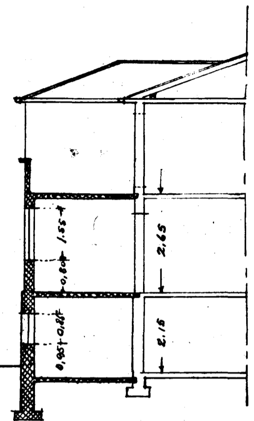
SKURÐUR A-B.
