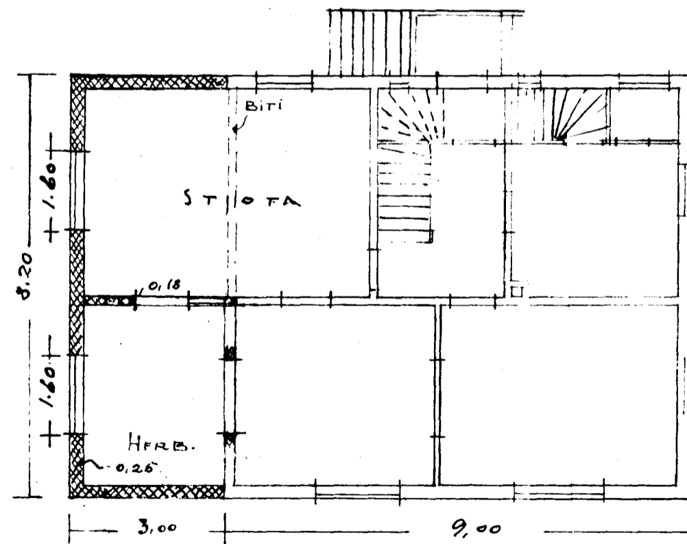
1. HÆÐ.
