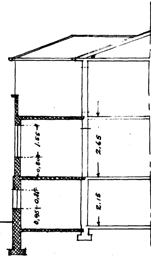
SKURÐUR A-B.
