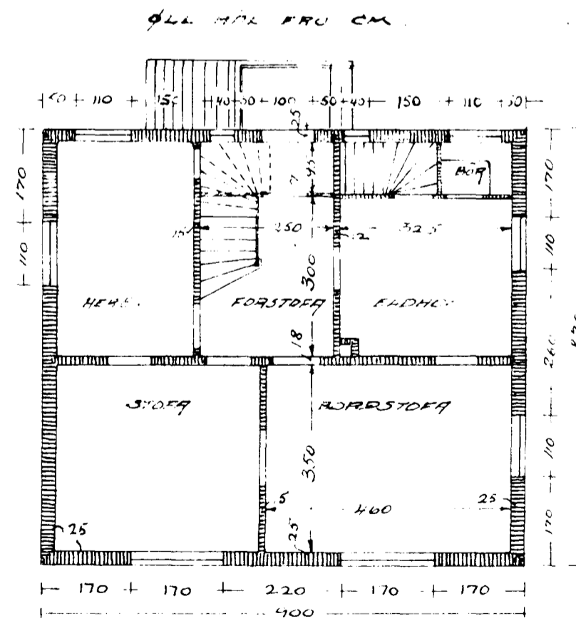
1. HÆÐ
