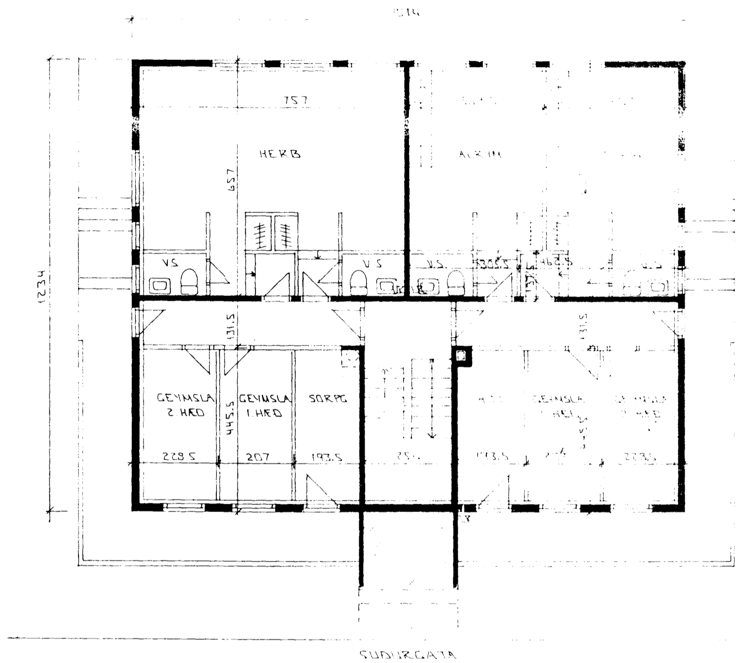
GRUNNMÝND JARÐHÆÐAR 1:100
