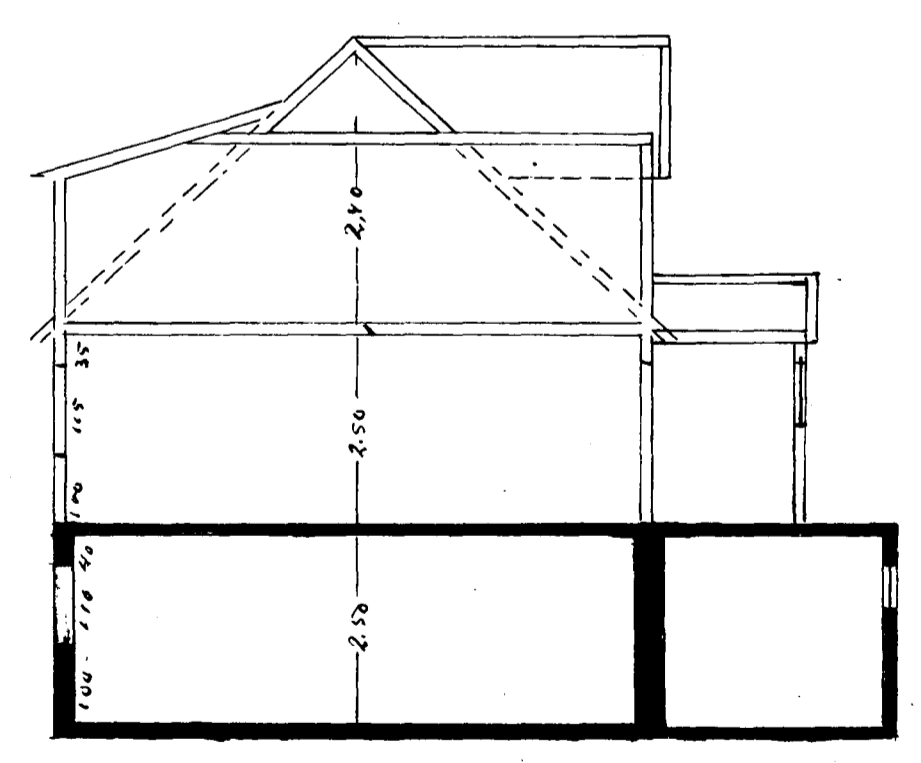
Skurður
