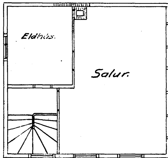
2. hæð.
