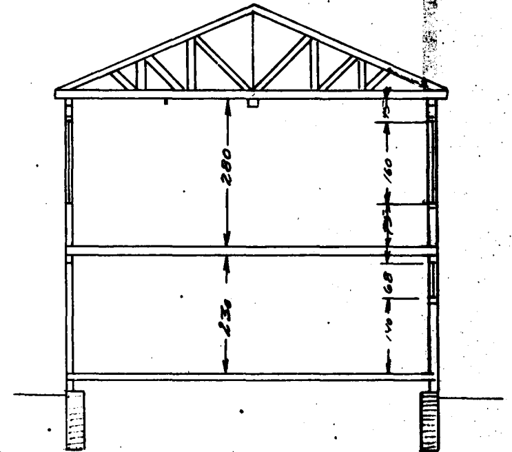
Þvershurður.
