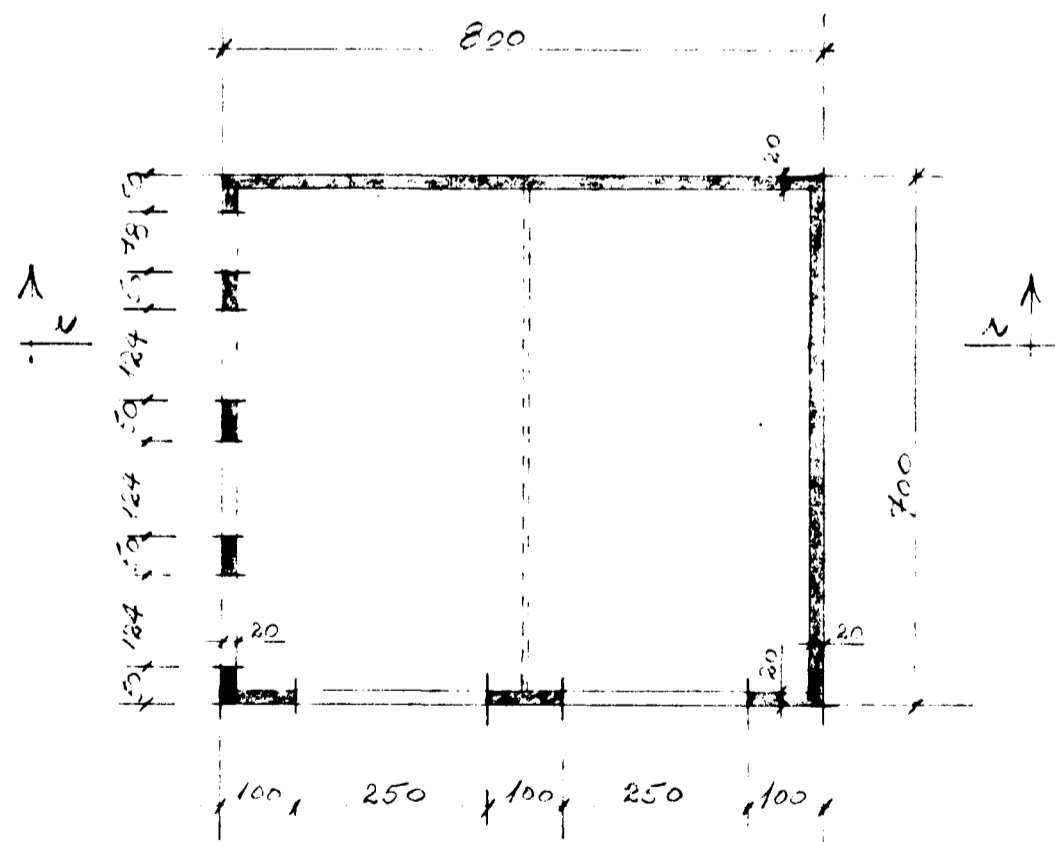
GRUNNMYND.
