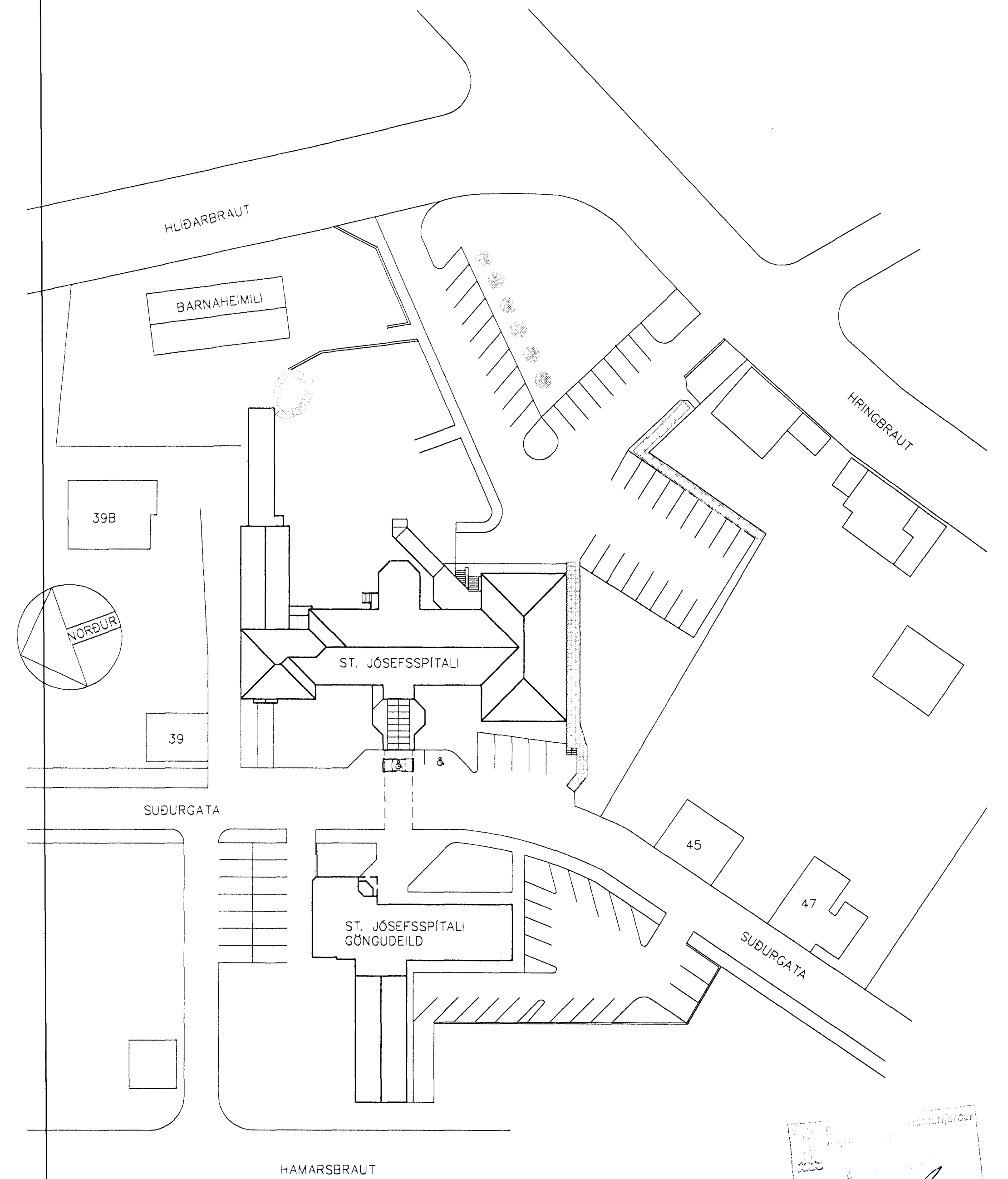
AFSTÖÐUMYND 1:500
