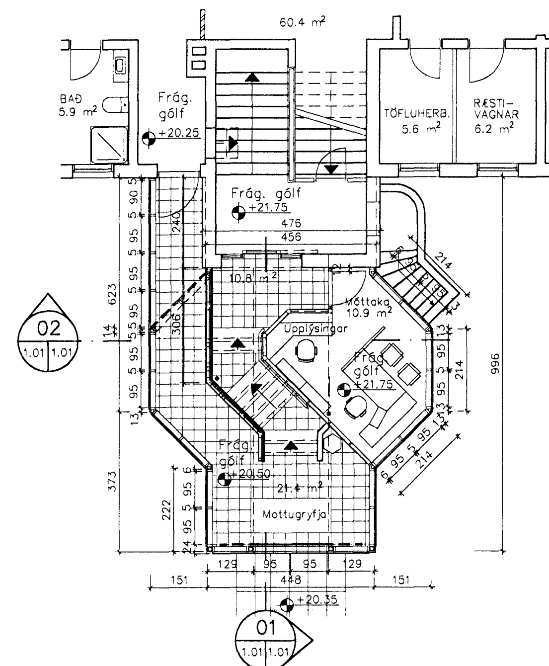
GRUNNMYND - ANDDYRISSKÁLI
