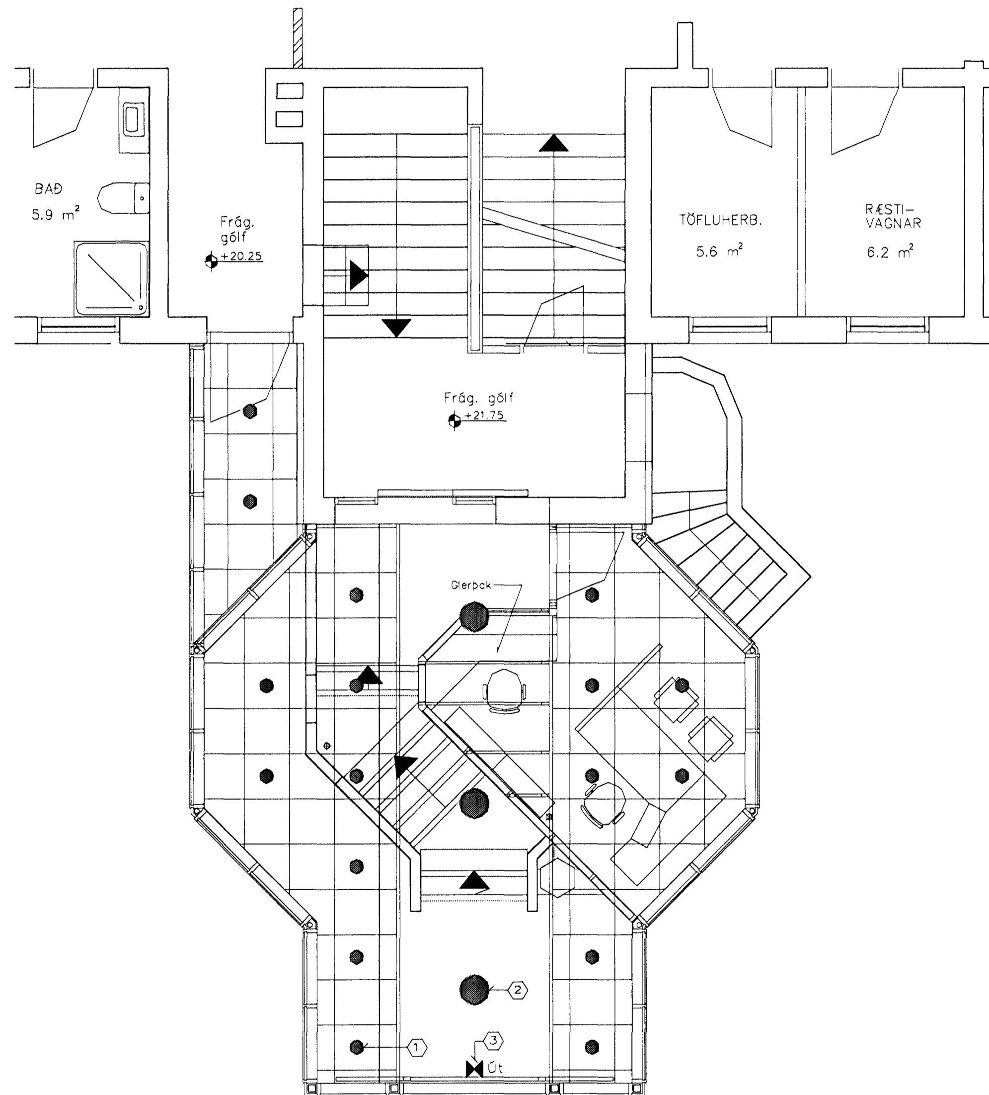
GRUNNMYND - LAMPAPLAN 1:50
