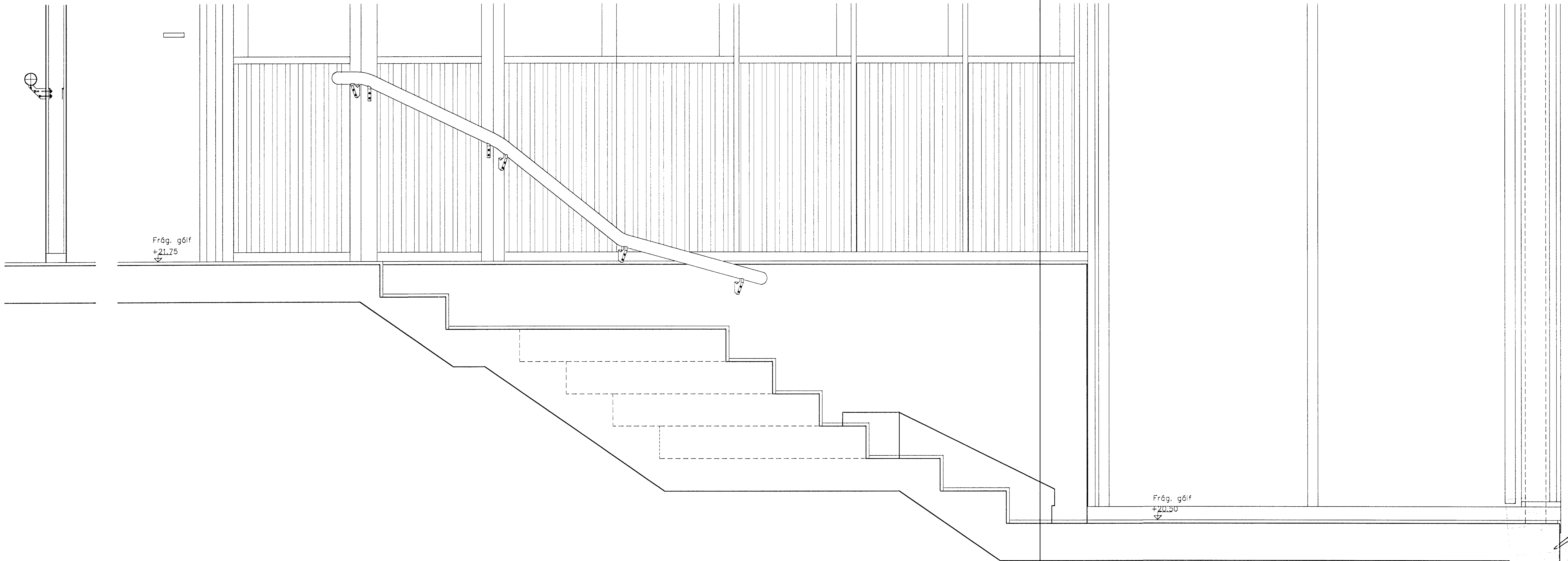
06 Snið 1:10 5.02/5.03
