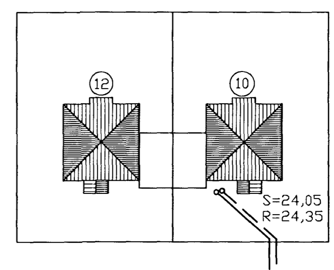
AFSTÖÐUMYND, 1:50
