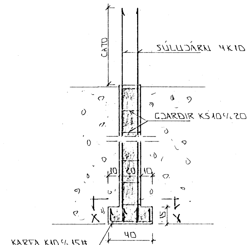
SÚLA S1 1:20
