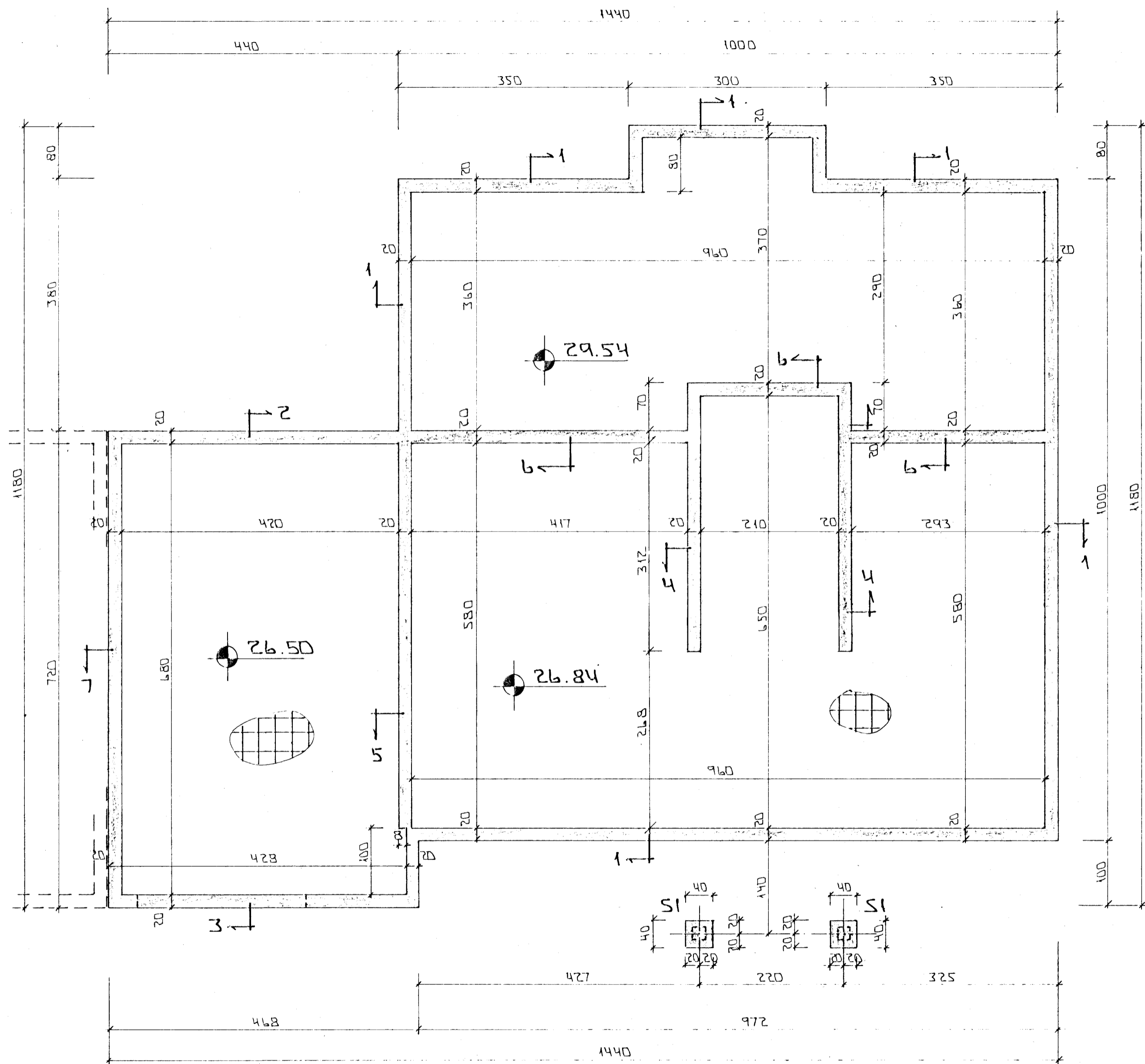
GRUNNMÝND 1:50
