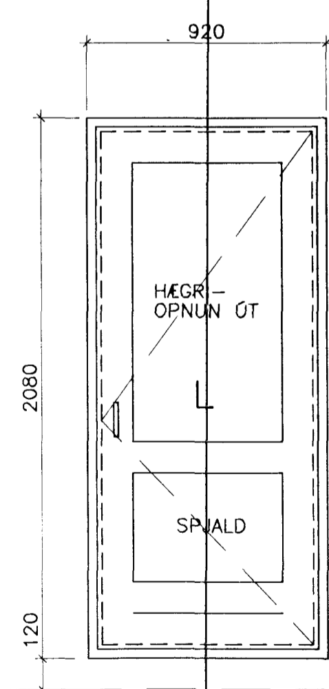
1 STK. HURD OPN. ÚT
