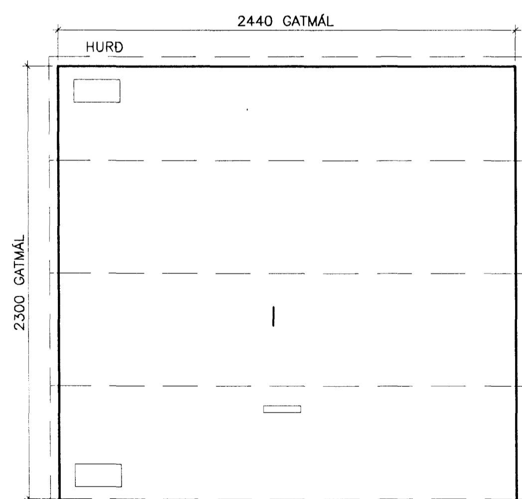
1 STK. BÍLGEYMSLUDYR, 2440X2300mm
