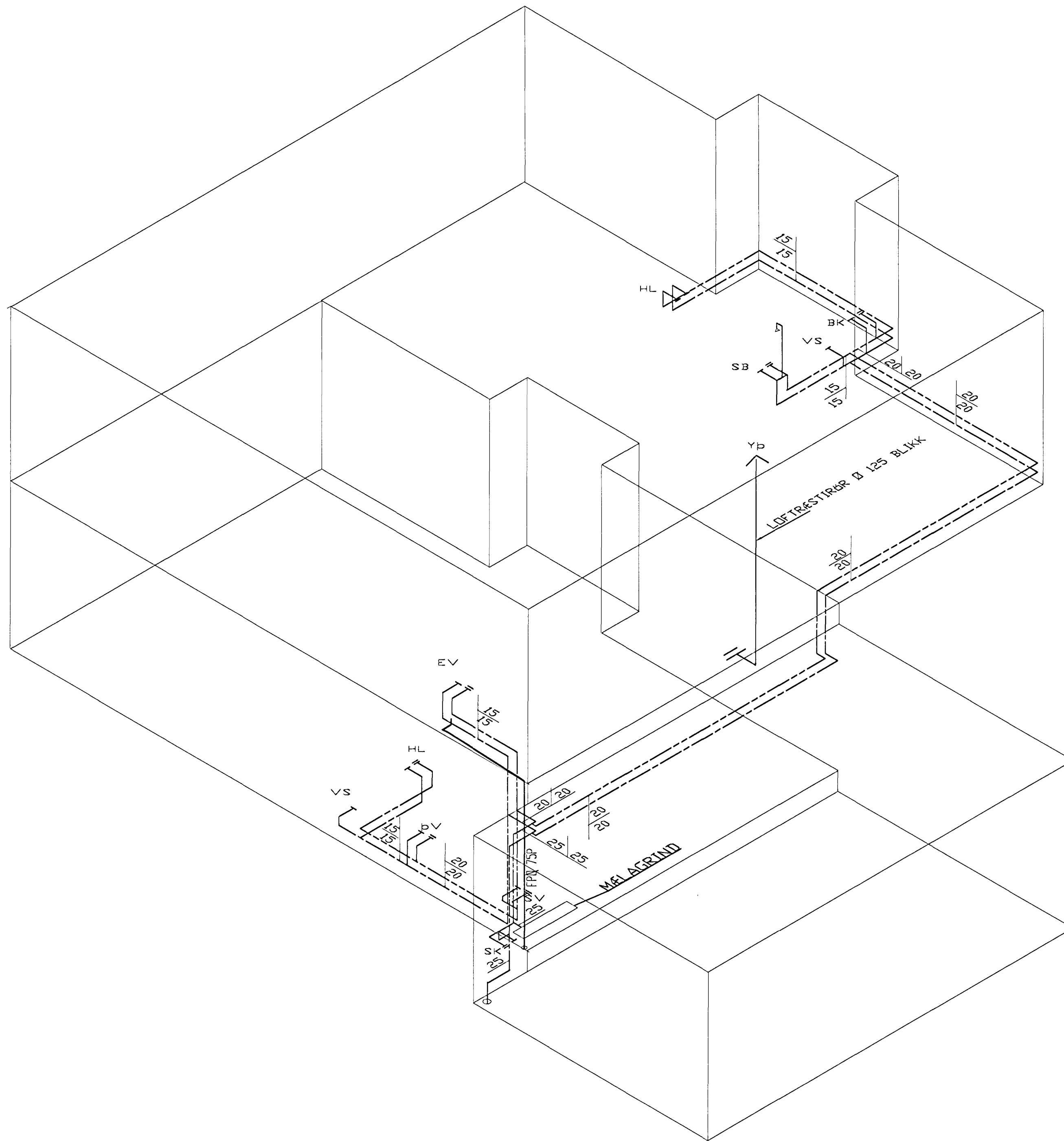
RÚMMYND VATNS OG FRÆRENNSLISLAGNA 1:50
