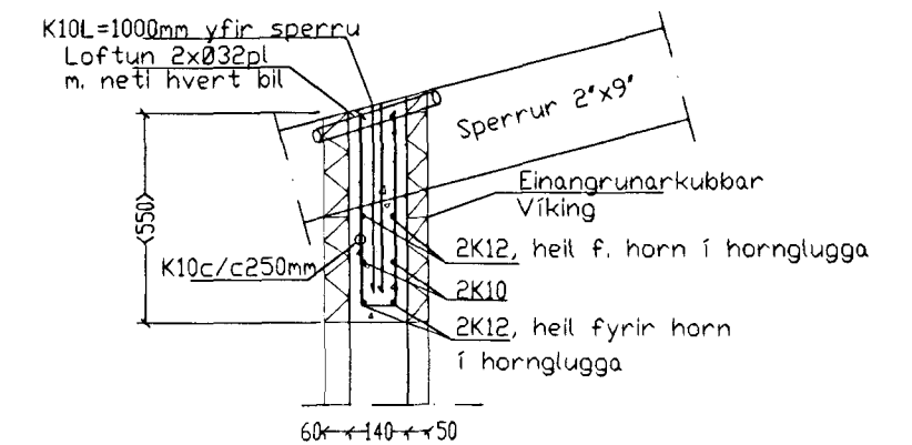
Snið C2 1:20
