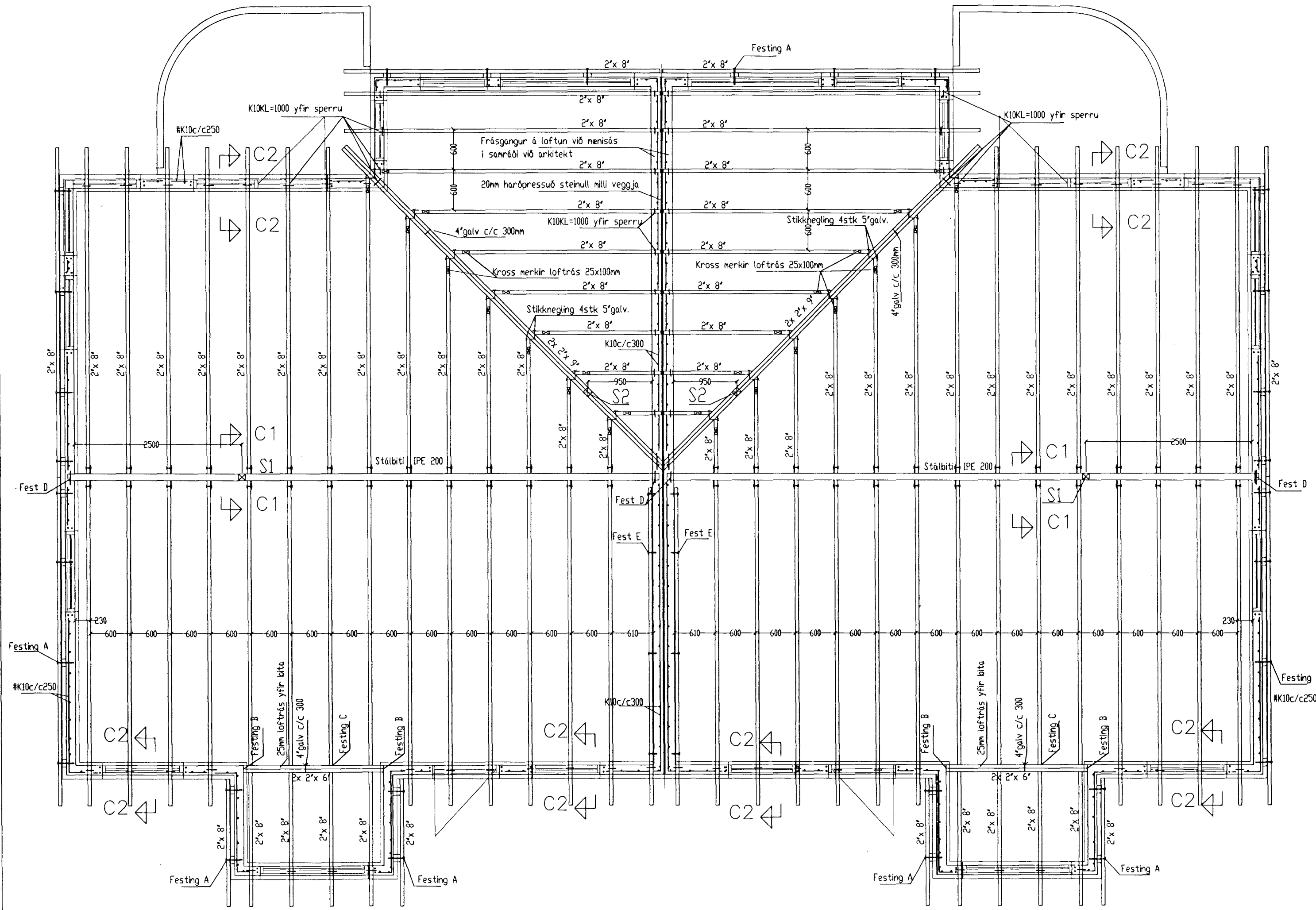
Grunnmynd þakvirkis 1:50
