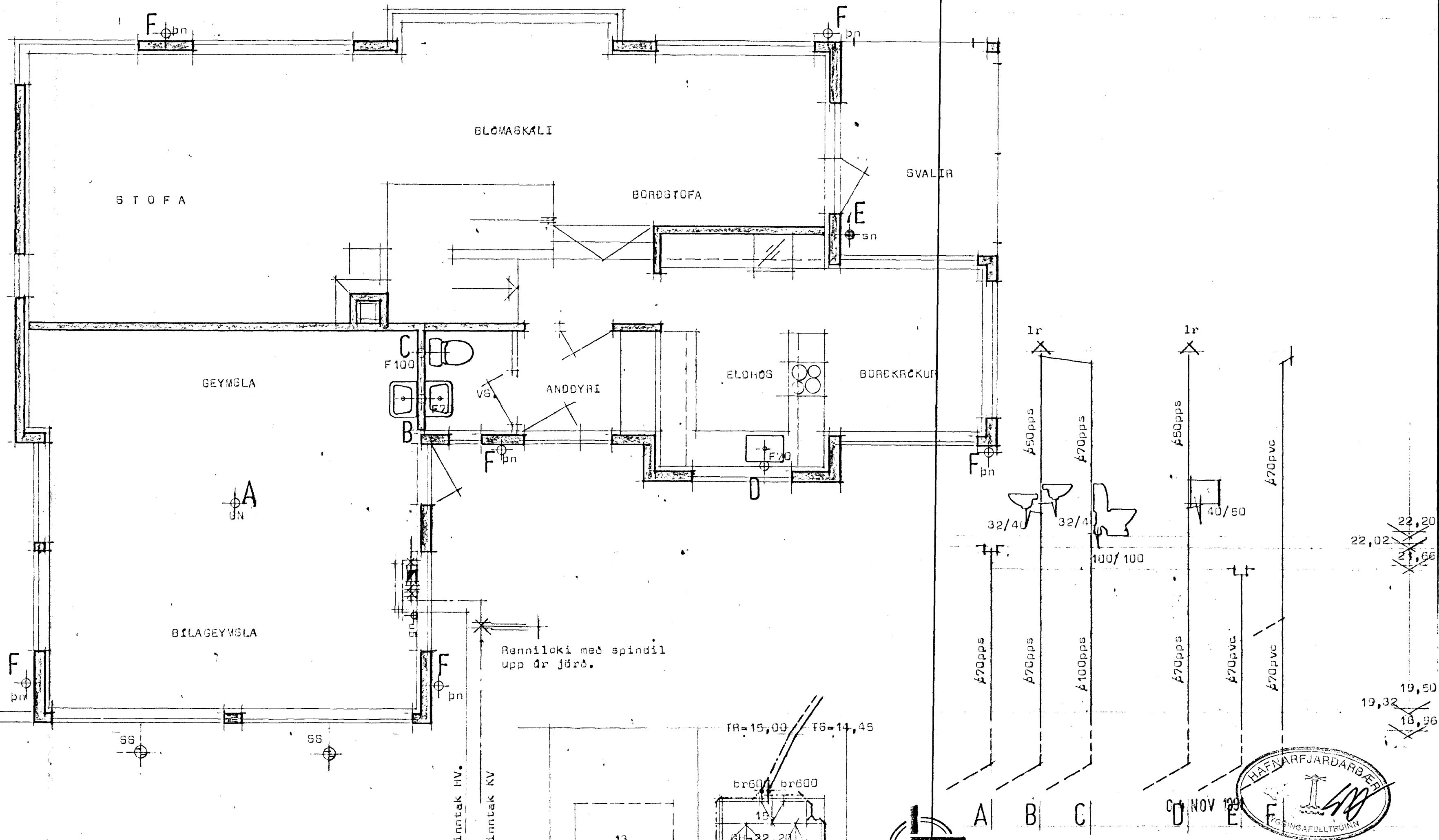
Grunnmynd afri hæðar MK 1:50
